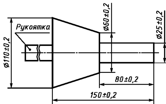
Рисунок 101 — Испытательный калибр
