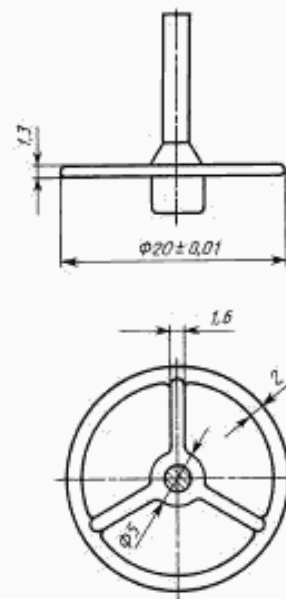
Рисунок 2 — Колесико мешалки с прорезями
