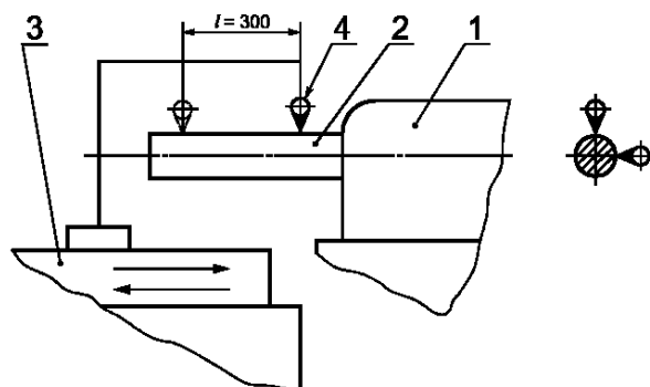
1 — задняя бабка; 2 — оправка; 3 — каретка; 4 — индикатор
