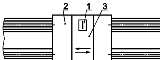
1 — уровень; 2 — каретка; 3 — шлифовальная бабка
