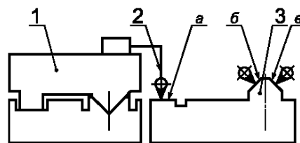
1 — каретка; 2 — индикатор; 3 — станина изделия
