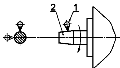
1 — индикатор; 2 — шпиндель
