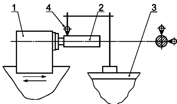
1 — шлифовальная бабка; 2 — контрольная втулка; 3 — станина изделия; 4 — индикатор
