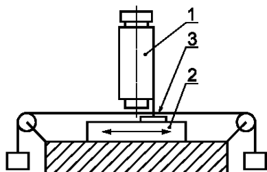
1 — микроскоп; 2 — каретка; 3 — натянутая струна
