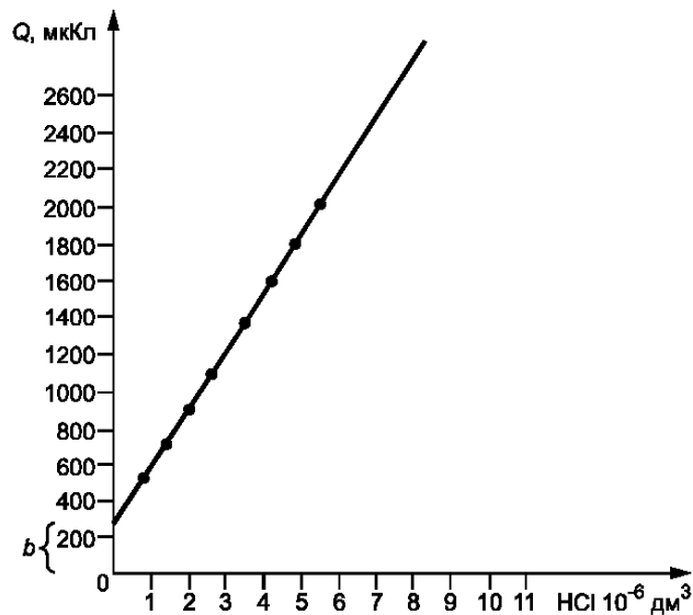
Рисунок 1 — Градуировочный график микрокулометра
