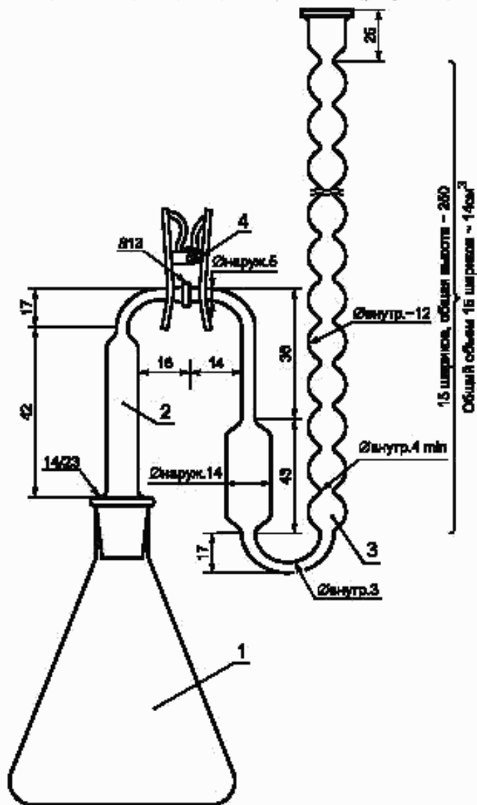
Рисунок 1 — Стеклянный прибор для отгонки и поглощения мышьяка
