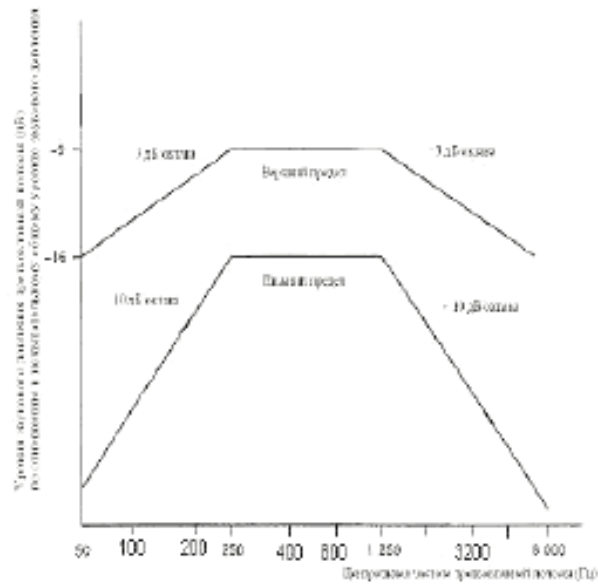
Рисунок 1 - Структура частотной характеристики для широкополосного шума
