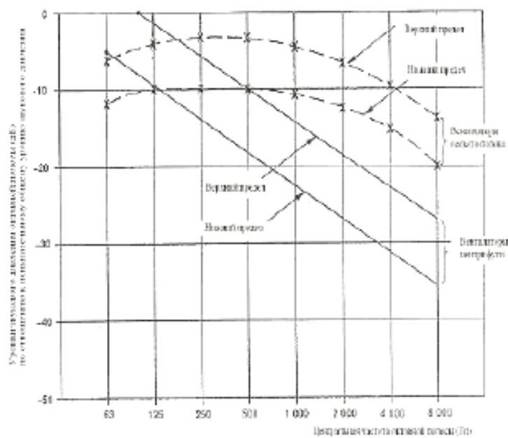
Рисунок 2 - Структура звуковой мощности для широкополосного шума (по [4], приложение В)
