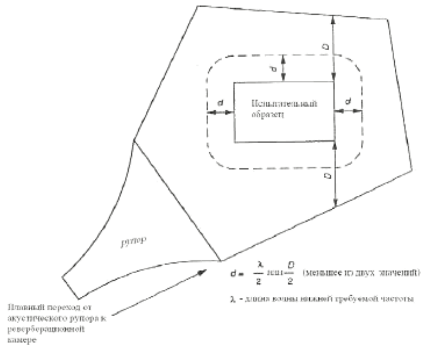
Рисунок 4 - Типовое расположение микрофонов вокруг образца
