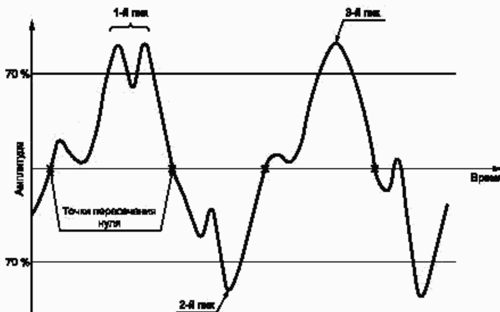
Рисунок 2 — Пример обнаружения пиков отклика, превышающих пороговое значение (70 %)
