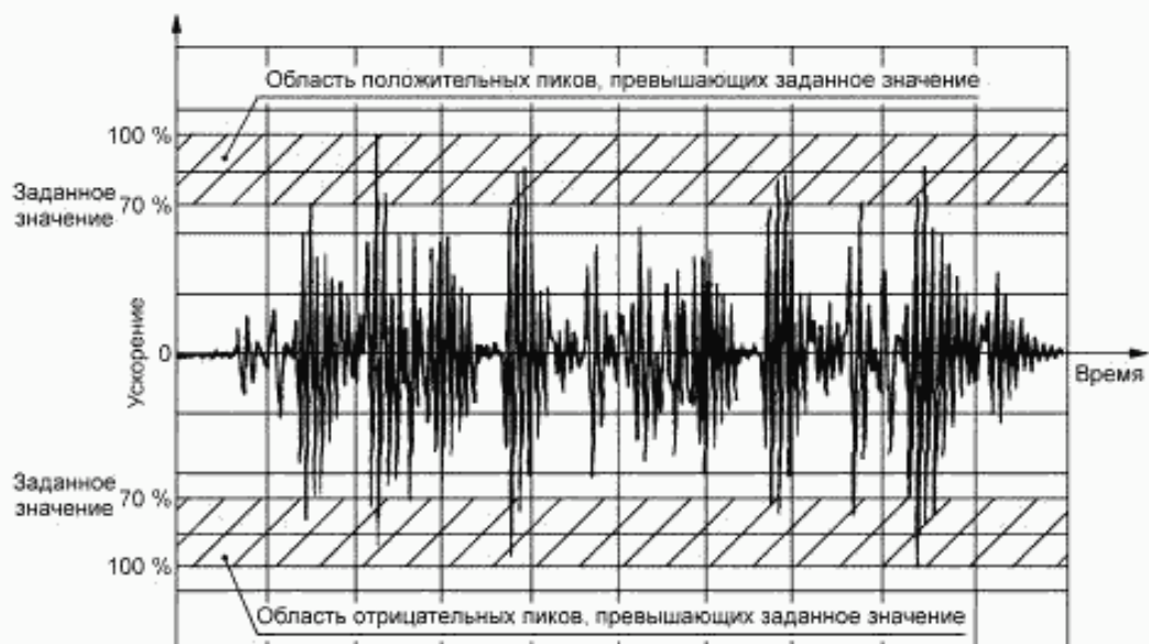
Рисунок 1 — Пример типичного отклика колебательной системы, возбуждаемой заданным временным процессом (пороговое значение 70 %)
