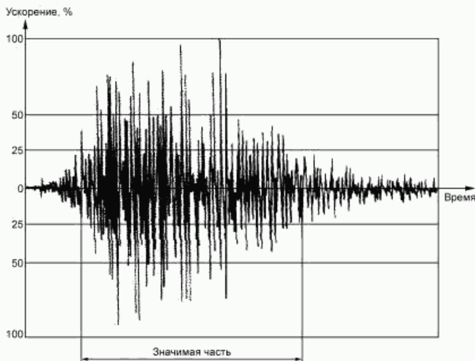
Рисунок 4 — Типичная форма акселерограммы
