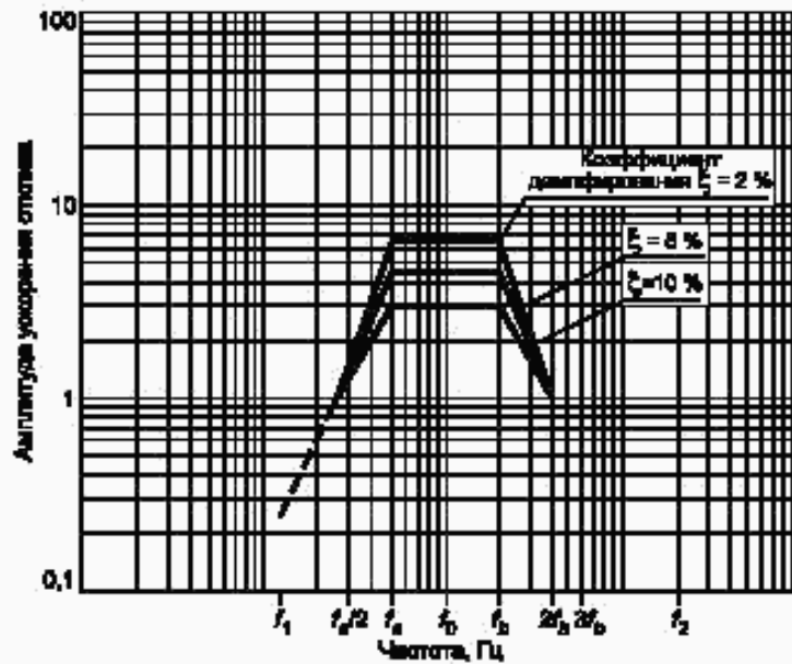
Рисунок — Категория 2. Рекомендуемый вид заданного спектра ответа
