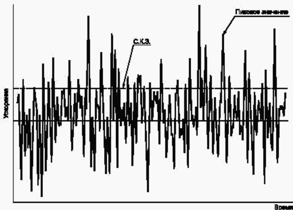
Рисунок A.2 — Отсечка (ограничение) сигнала
