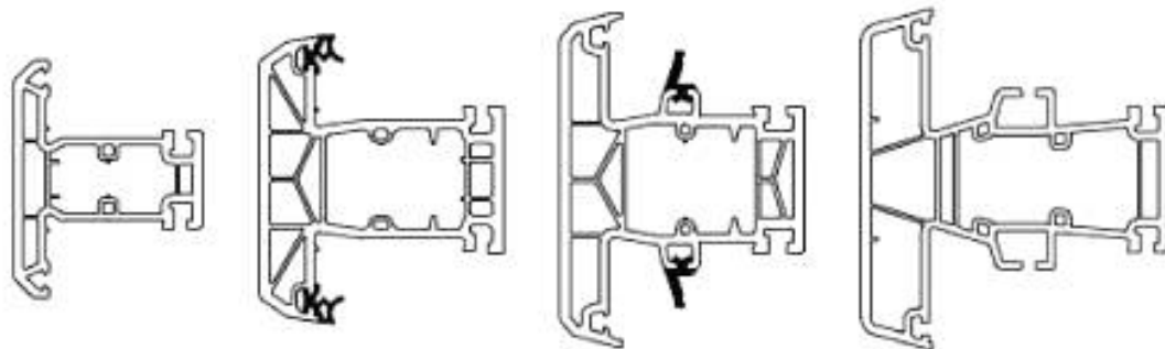
Сечения профилей импостов
