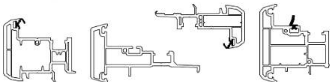
Сечения профилей ступцов
