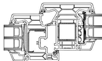
в) Импостный притвор с одной открывающейся створкой
