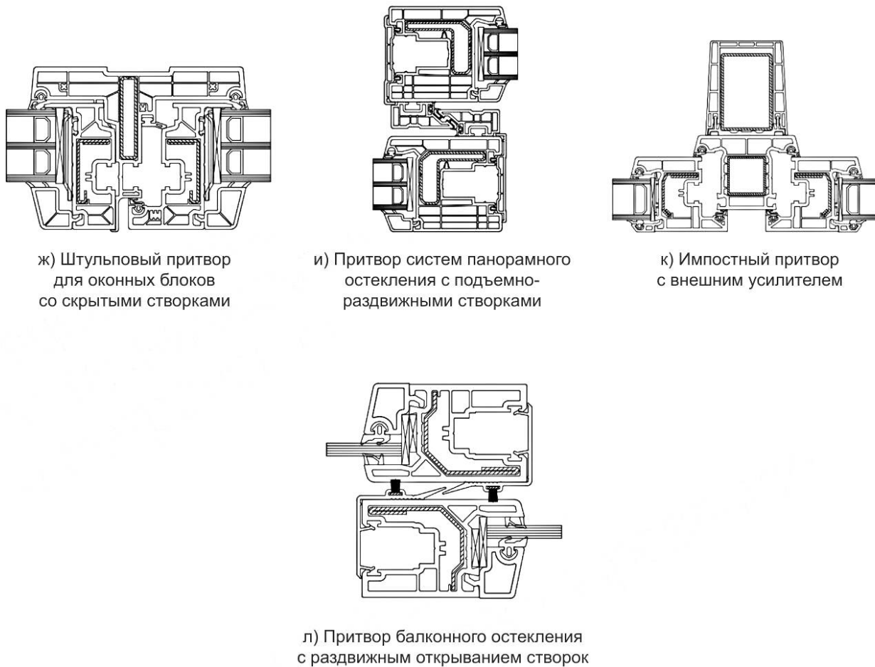
Рисунок 2 — Примеры импостного и штупельного притворов оконных и балконных блоков
