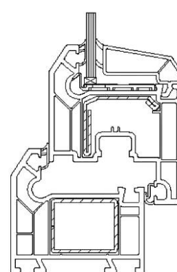
и) Балконный дверной блок из четырехкамерных профилей с поворотным и поворотно-откидным открыванием створки
