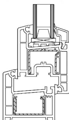
а) Оконный блок из трехкамерных профилей
