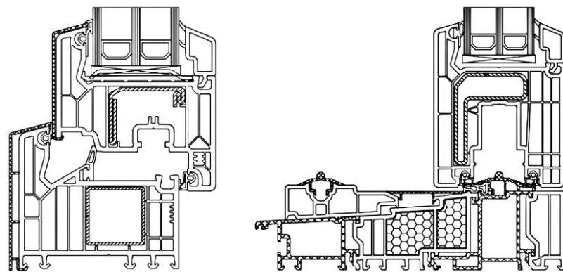
к) Оконный блок из многокамерных профилей с декоративными алюминиевыми накладками
