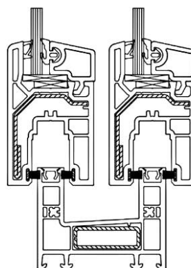
ж) Балконное остекление из однокамерных профилей с раздвижным открыванием створок
