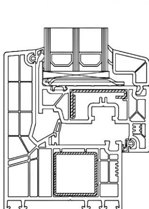
д) Оконный блок со скрытой створкой из многокамерных профилей
