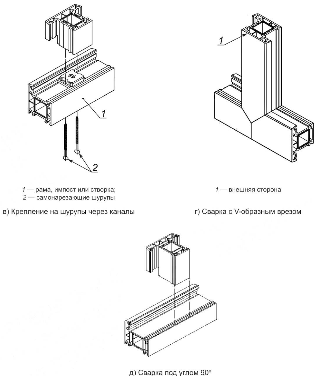
Рисунок 4 — Примеры крепления импостов
