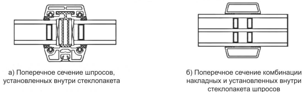
Рисунок 6 — Варианты установки декоративных раскладок
