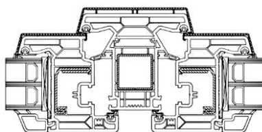
б) Импостный притвор с двумя открывающимися створками для оконных блоков с декоративными алюминиевыми накладками
