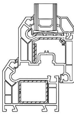
б) Оконный блок из четырехкамерных профилей
