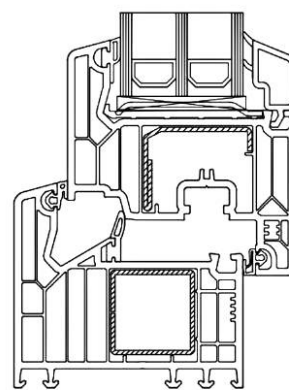
г) Оконный блок со створкой из шестикамерного и коробкой из семикамерного профилей
