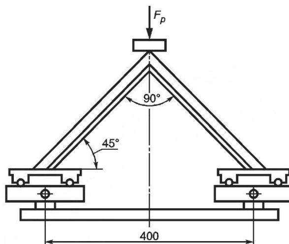
F_p — вертикальная сжимающая нагрузка на угловое соединение Рисунок 11 — Схема Б приложения разрушающей нагрузки F_p при определении прочности угловых соединений
