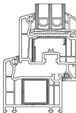
в) Оконный блок из пятикамерных профилей
