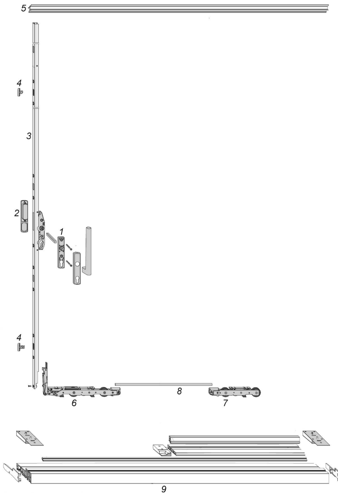
1 — ручка в наборе; 2 — внешняя ручка; 3 — привод; 4 — запорная планка; 5 — направляющая верхняя шина; 6 — ведущая каретка; 7 — ведомая каретка; 8 — соединительная тяга; 9 — направляющая нижняя шина в наборе
