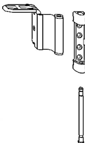
Рисунок В.6 — Верхняя петлевая группа
