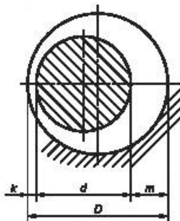
Рисунок 17 — Соединение с плавающими втулками
