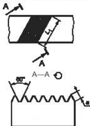
Рисунок Б.1 — Пример взрывозащитной поверхности щелевого огнепреградителя разгрузочного устройства с канавками сечением в виде равнобедренного треугольника
