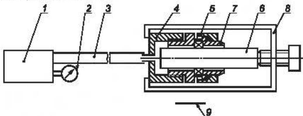
1 — гидравлический насос; 2 — манометр; 3 — гибкий шланг; 4 — приспособление для подсоединения; 5 — испытуемое уплотнительное кольцо; 6 — вал из мягкой стали; 7 — зажимающее кольцо; 8 — крепящая обойма; 9 — бумага.
