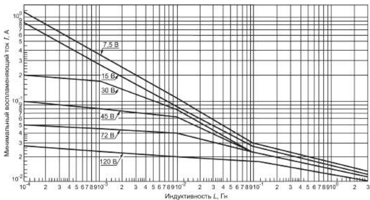
Рисунок А.10 — Индуктивные цепи подгруппы IIC
