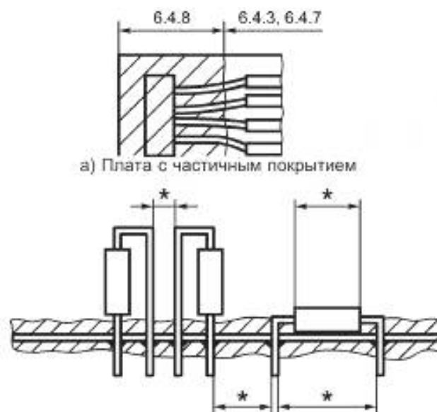
б) Плата с пайкой выступающих выводов резисторов
