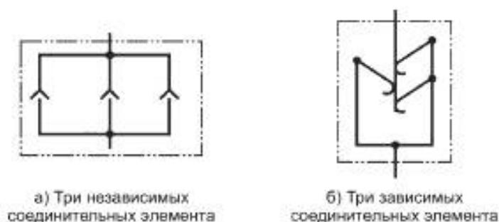
Рисунок 2 — Примеры автономных и неавтономных соединительных элементов
