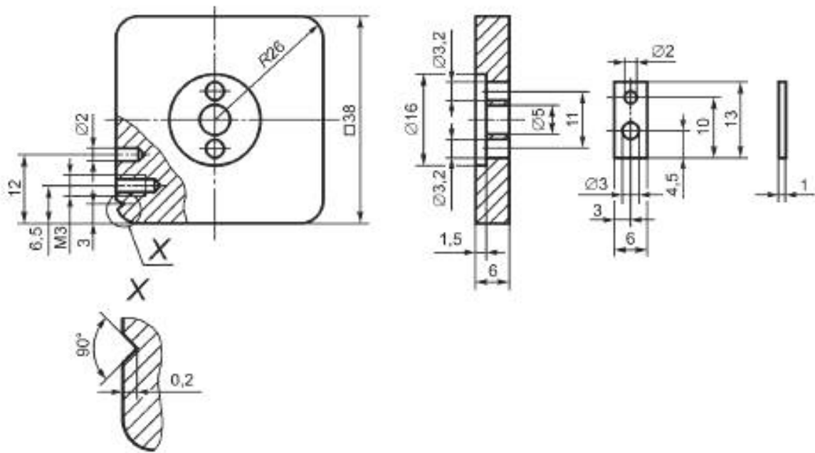
Рисунок Б.3 — Держатель проволошек
