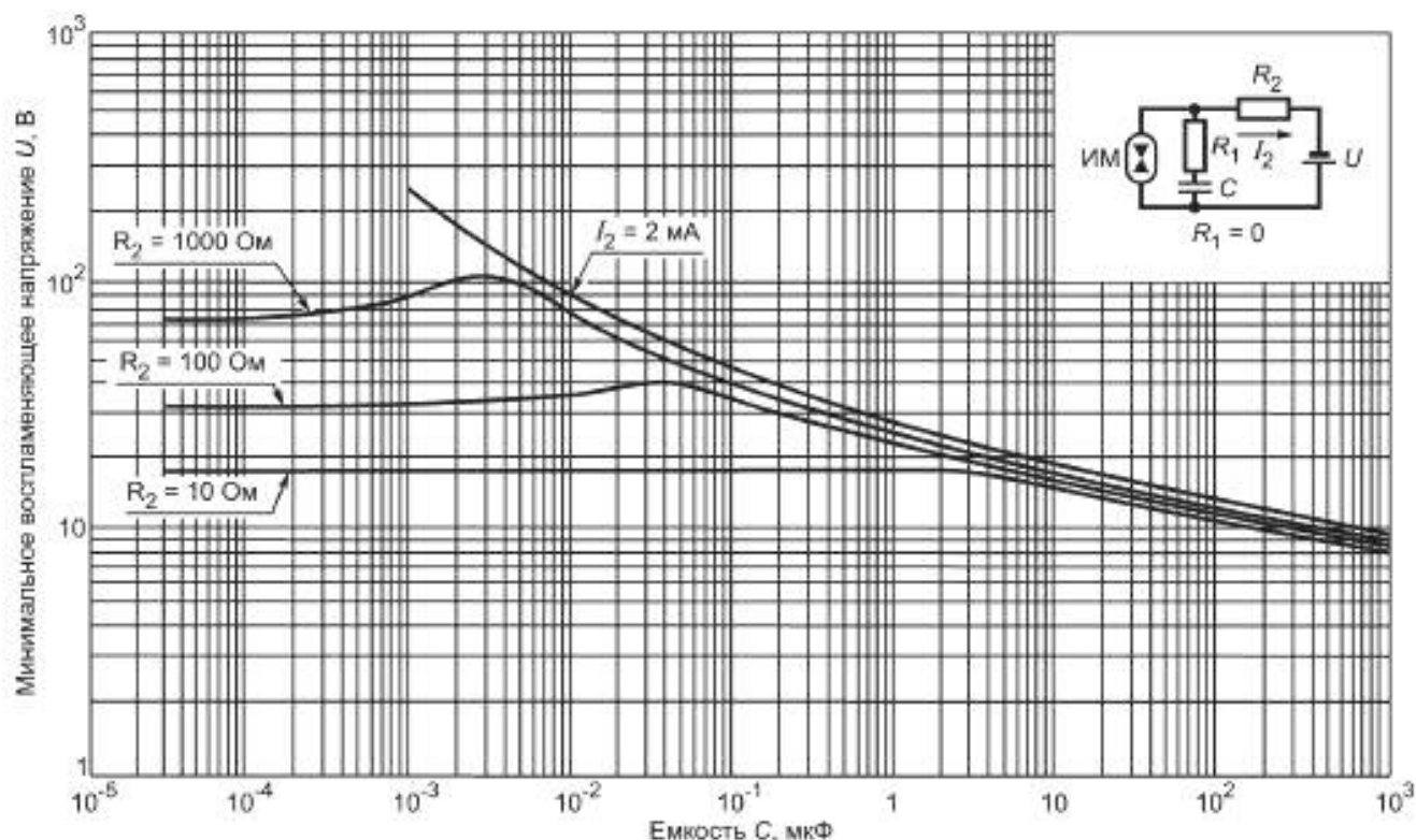
Рисунок А.12 — Минимальное воспламеняющее напряжение в активизированной взрывоопасной водородно-кислородной смеси (81 % H_2 + 19 % O_2 ) для емкостных цепей подгруппы IIА при R_1 = 0 \text{ Ом}
