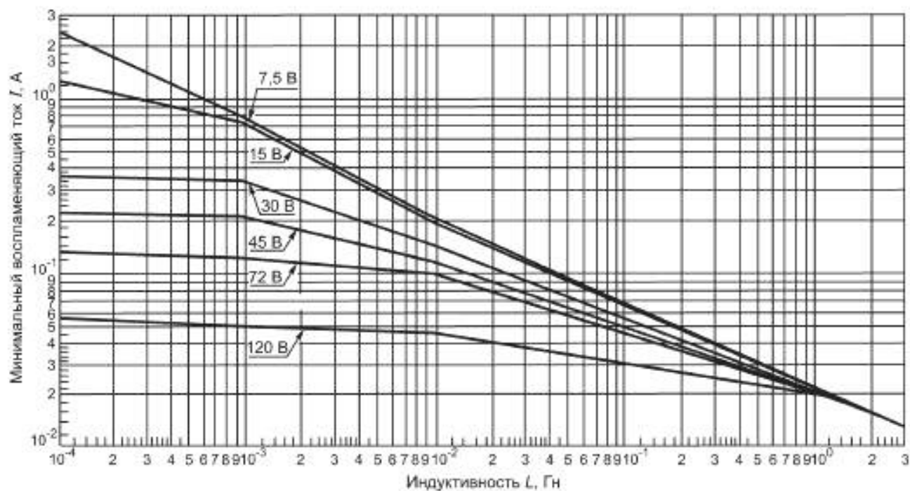
Рисунок А.9 — Индуктивные цепи подгруппы IIB
