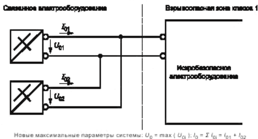
Рисунок В.2 – Параллельное соединение. Суммирование токов
