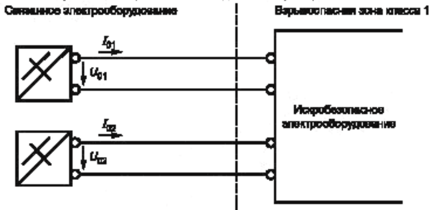
Рисунок В.3 – Последовательные и параллельные соединения. Суммирование напряжений и токов
