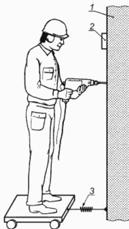
1 — бетонная стена; 2 — устройство считывания силы нажатия; 3 — динамометр
