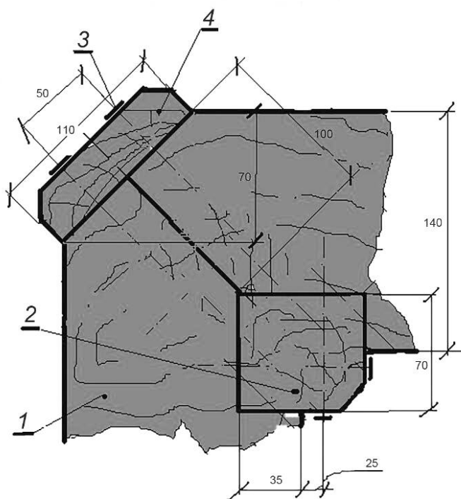
Рисунок В.3 — Брус стеновой 100×140 мм со шпонкой 70×70 мм и нащельником 30×110 мм (оба на всю высоту стены)
