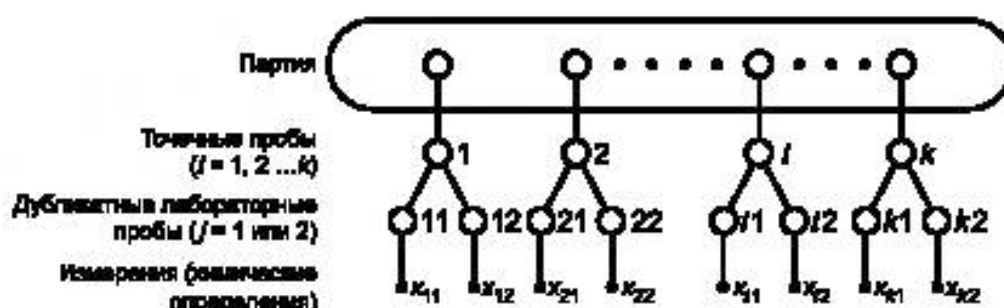
Рисунок 1 — Схема, применяемая к легкодробимым ферросплавам (вид I)
