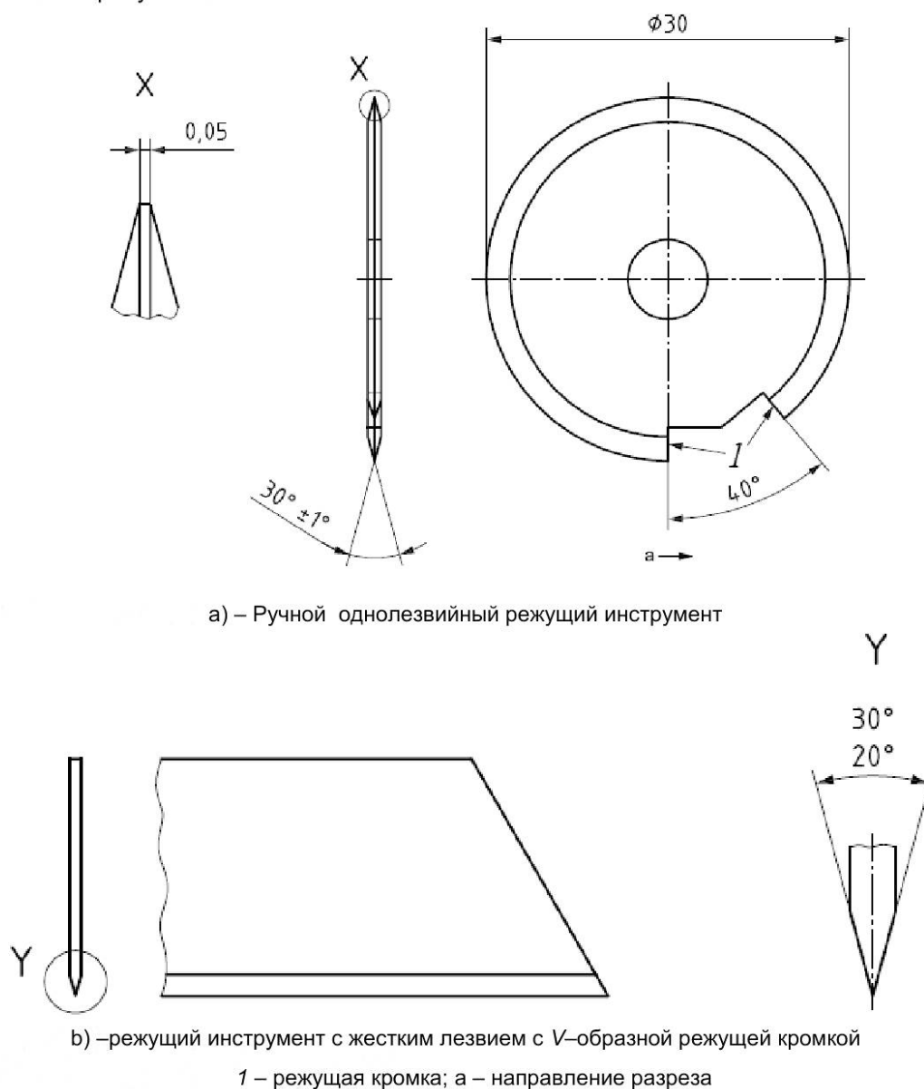
Рисунок 1 – Однолезвиевые режущие инструменты
