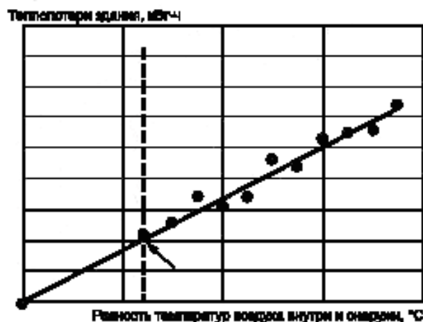
Рисунок 1 — Схема функциональной зависимости тепловых потерь здания от разности температур воздуха внутри и снаружи
