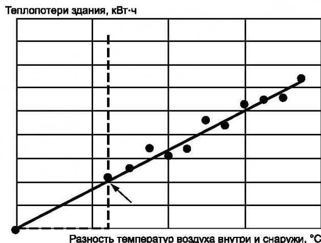
Стрелкой отмечены суммарные тепловыделения в помещениях здания
