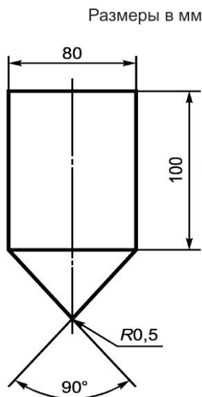
Рисунок 6 — Испытательный конус
