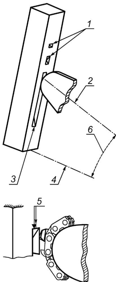
1 — неучитываемые пропилы; 2 — центральная ось направляющей шины; 3 — пропил; 4 — горизонталь; 5 — угол выхода из цепи образца измеряют в самой верхней точке площади пропила, не обращая внимания на другие возможные пропилы, 6 — угол выхода из образца
