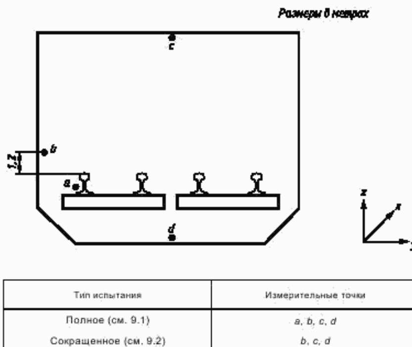
Рисунок 1 — Измерительные точки в плане поперечного сечения туннеля в зависимости от типа испытаний
