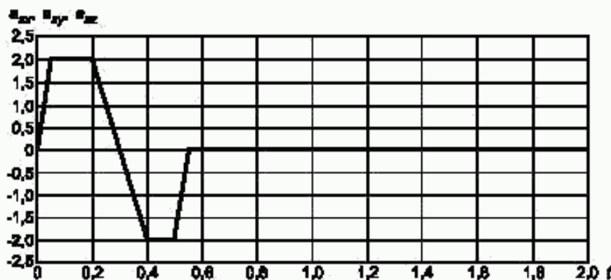
а) Входной сигнал ускорения на подушке сиденья
