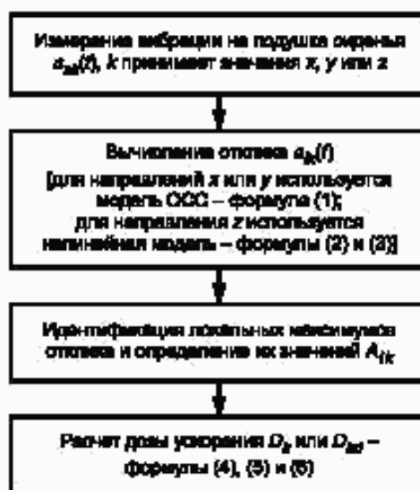
Рисунок 1 — Блок-схема расчета дозы ускорения
