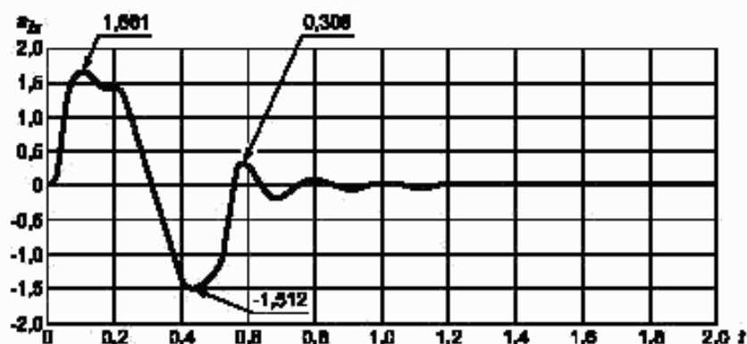
c) Реакция позвоночника в направлении z
