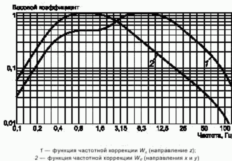
Рисунок В.1 — Функции частотной коррекции W_x и W_z для определения параметров общей вибрации
