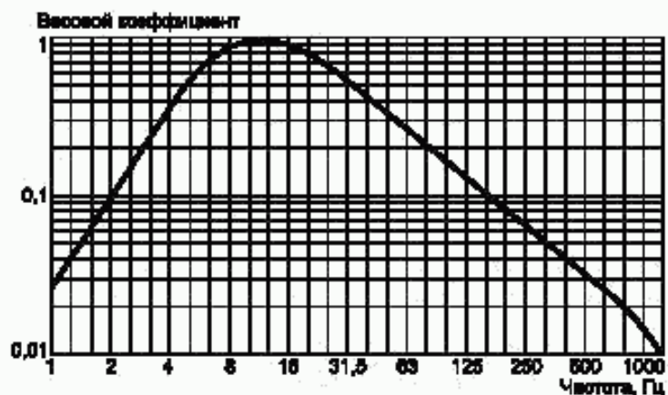
Рисунок В.2 — Функция частотной коррекции W_b для определения параметров локальной вибрации
