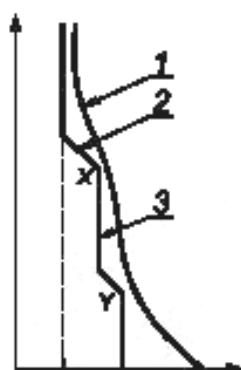
1 — преддугловая характеристика; 2 — прямая постоянного значения I^2t ; 3 — условная кривая перегрузок
