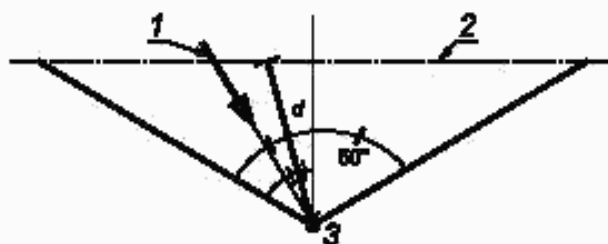
1 — среднее направление ветра; 2 — осевая линия дороги; 3 — микрофон
