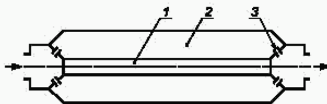
1 — входной канал; 2 — кольцевая полость; 3 — дроссельные устройства (лопастные вставки или отверстия малого диаметра)
