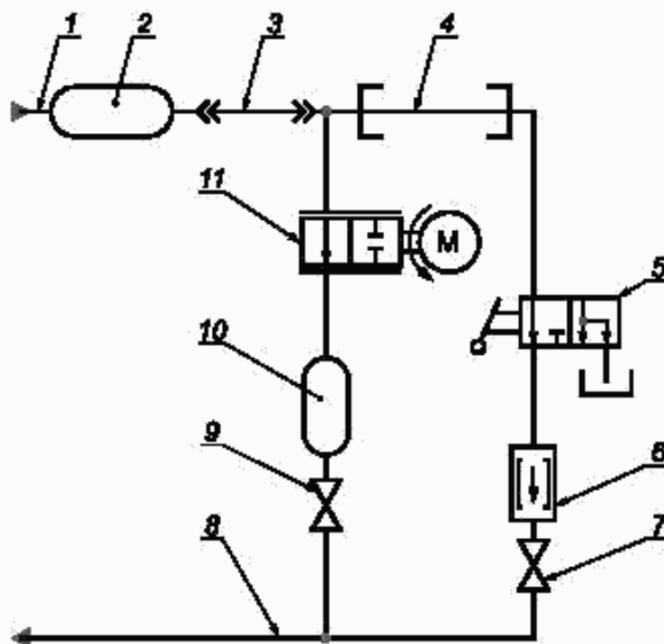
1 — магистраль нагнетания жидкости от насосной станции; 2, 10 — баллон блока акустической развязки; 3 — трубопровод с суженным диаметром проходного сечения; 4 — очищаемая магистраль трубопровода; 5 — пробоотборник; 6 — гаситель колебаний давления жидкости; 7, 9 — регулирующий вентиль; 8 — магистраль слива в насосную станцию; 11 — генератор колебаний жидкости
