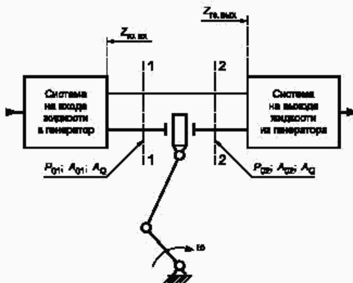
Рисунок В.1 — Схема гидравлической цепи с генератором колебаний жидкости
