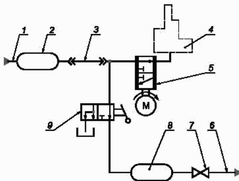
Рисунок 4 — Схема пульта для гидродинамической очистки проточных агрегатов
