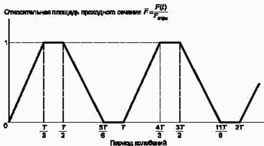
Рисунок В.2 — График зависимости площади проходного сечения для потока мощней жидкости от времени при работе генератора колебаний жидкости
