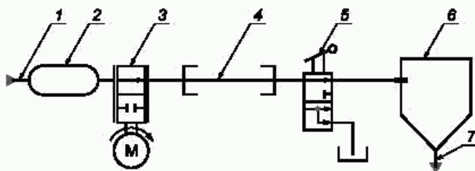
Рисунок 1 — Схема пульта для гидродинамической очистки трубопроводов в состоянии поставки
