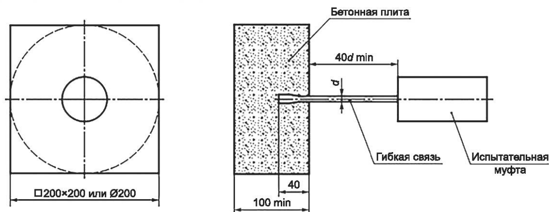
а) Образец с прямолинейной композитной гибкой связью
