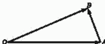
Рисунок G.1 — Векторный эффект установки пробных масс
