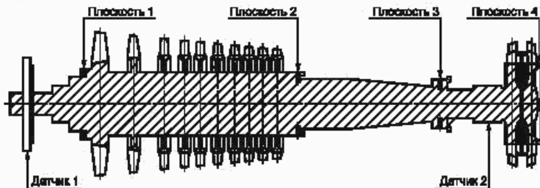
Рисунок D.1 — Ротор турбины
