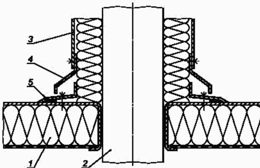
1 — потолочная панель; 2 — выхлопная труба; 3 — облицовка теплоизоляции; 4 — collar; 5 — резиновое уплотнение Рисунок А.16 — Пример акустической защиты отверстия в потолке с теплоизоляцией
