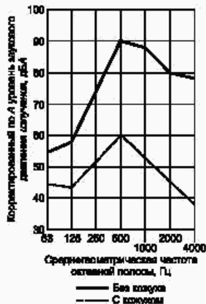
Рисунок 3 — Типичный пример корректрированных по А октавных уровней звукового давления излучения до и после установки кожуха
