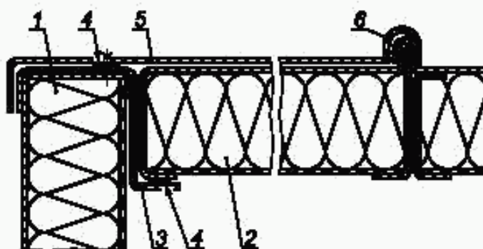
1 — стенка; 2 — потолочная панель; 3 — несущий профиль; 4 — резиновое уплотнение; 5 — защищающая от осадков кровля; 6 — защищающий от осадков кожух
