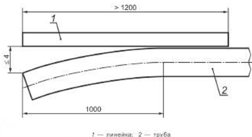
Рисунок 2 — Измерение концевой прямолинейности
