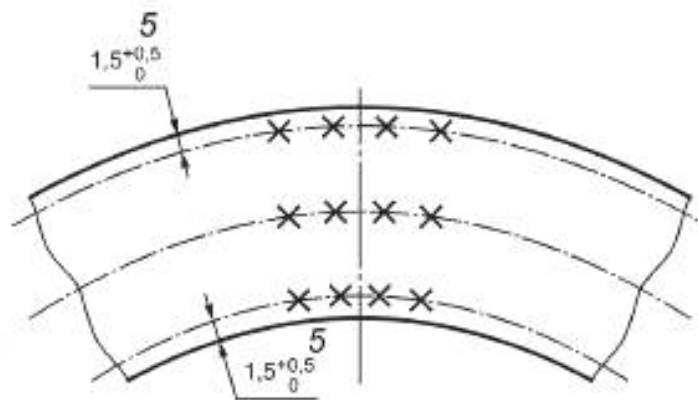
а — Бесшовная труба
