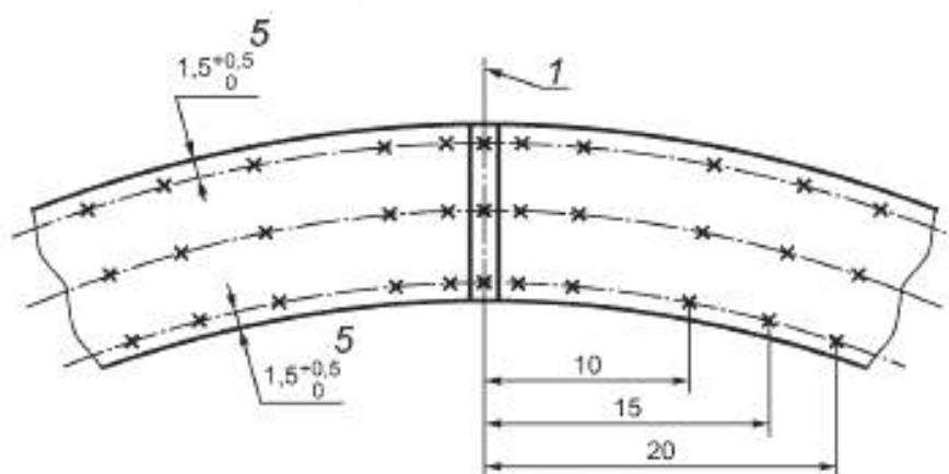
в — Труба ВЧС
