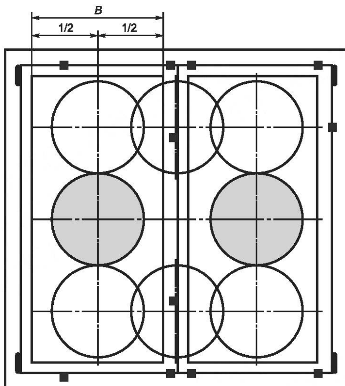
Рисунок Г.2 — Точки приложения динамических нагрузок на двустворчатом оконном блоке
