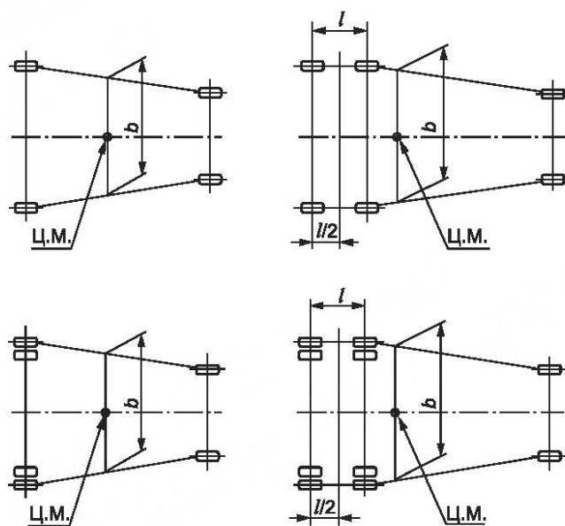
Рисунок 1 — Схемы определения величины приведенной колеи b
