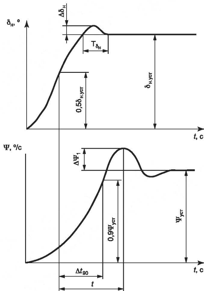
Рисунок 4 — Записи угла поворота рулевого колеса \delta_n и угловой скорости \psi АТС при испытании «рывок руля»
