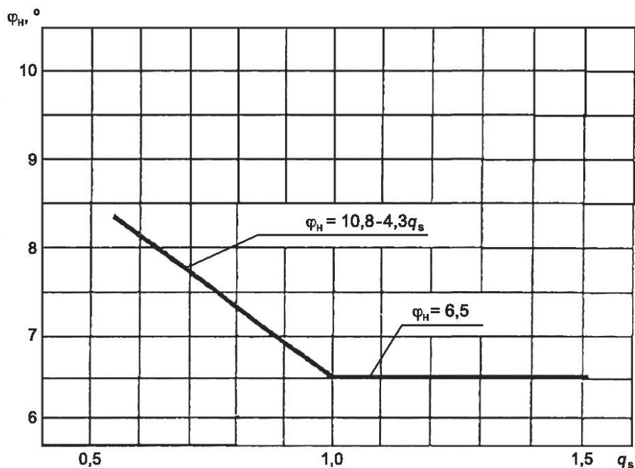
Рисунок 3 — Зависимость угла крена \varphi_H поддресоренных масс АТС от коэффициента поперечной устойчивости q_s
