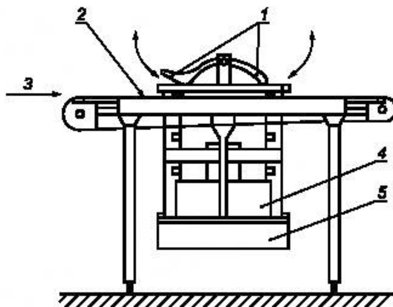
Рисунок 1 — Напольная пила
