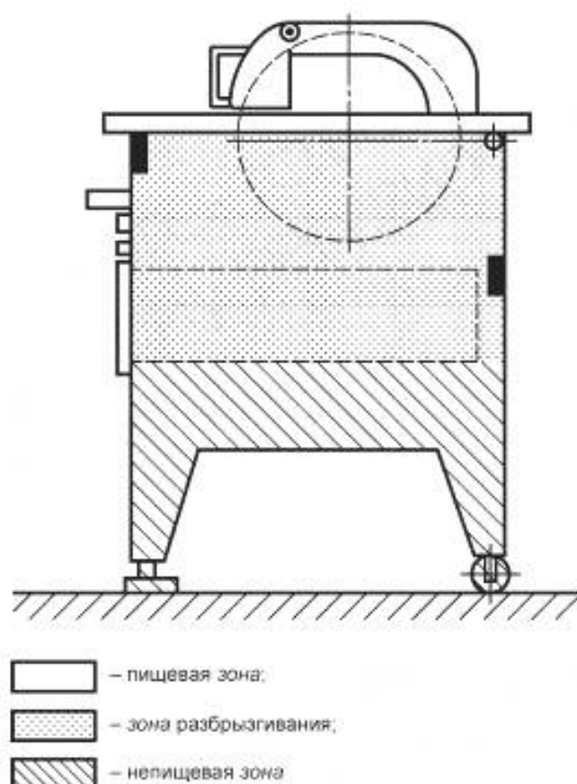
Рисунок 10 — Гигиенические области в пилах
