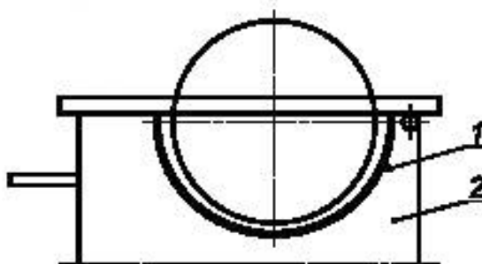
1 — фиксированная защита; 2 — закрытый корпус пилы
