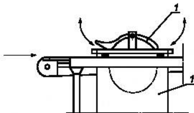
Рисунок 7 — Защитный кожух
