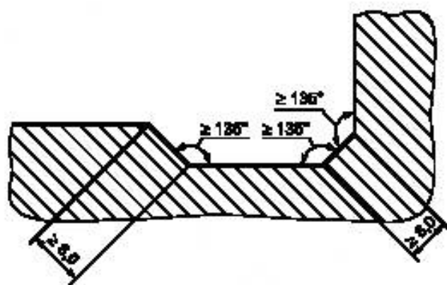
Рисунок А.3 — Углы в пищевой зоне
