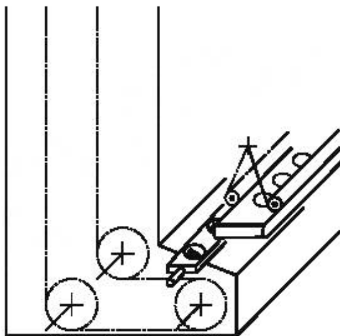
Рисунок 12 — Выталкивающее устройство
