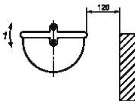
Рисунок 5 — Промежуток между неподвижным краем и осью крепления льюшек
