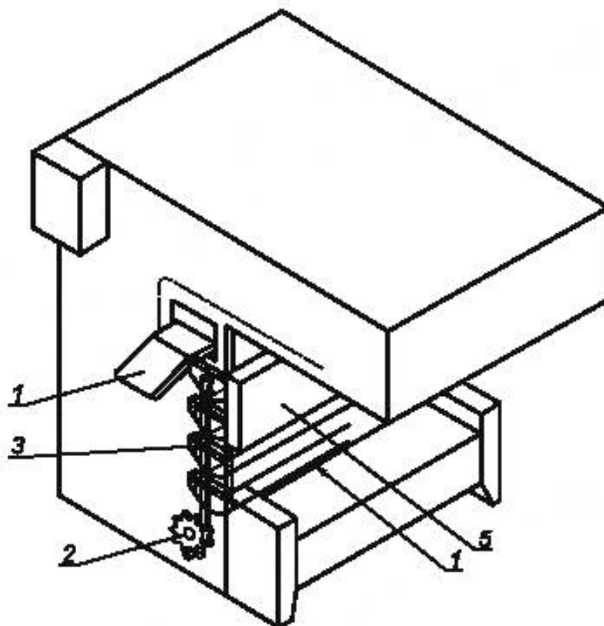
Рисунок 1— Загрузка тестовых заготовок спереди, боковая разгрузка
