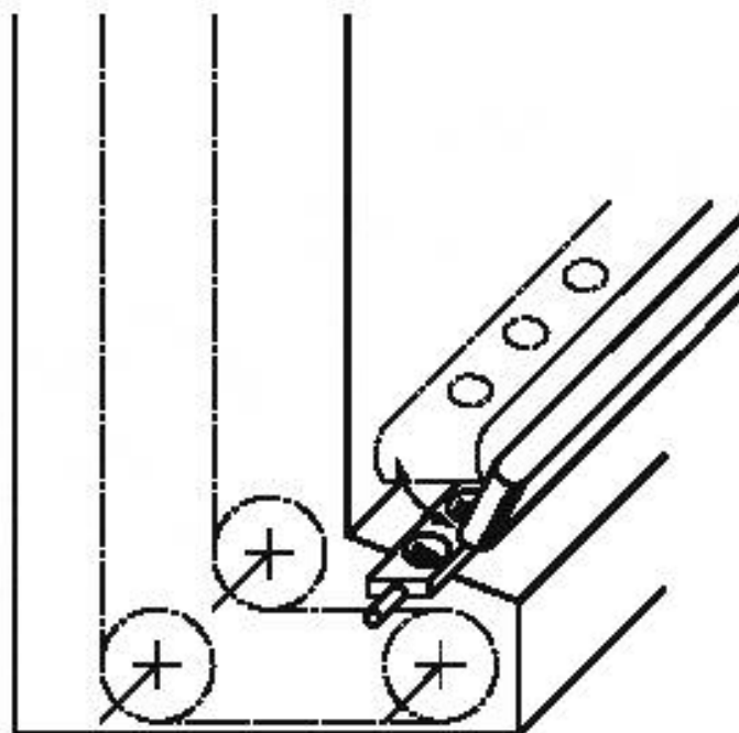
Рисунок 10 — Простов наклоняющее устройство
