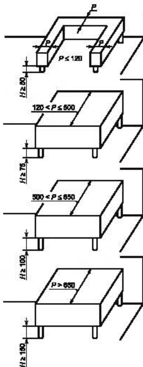
Рисунок А.18 – Станины для шкафов
