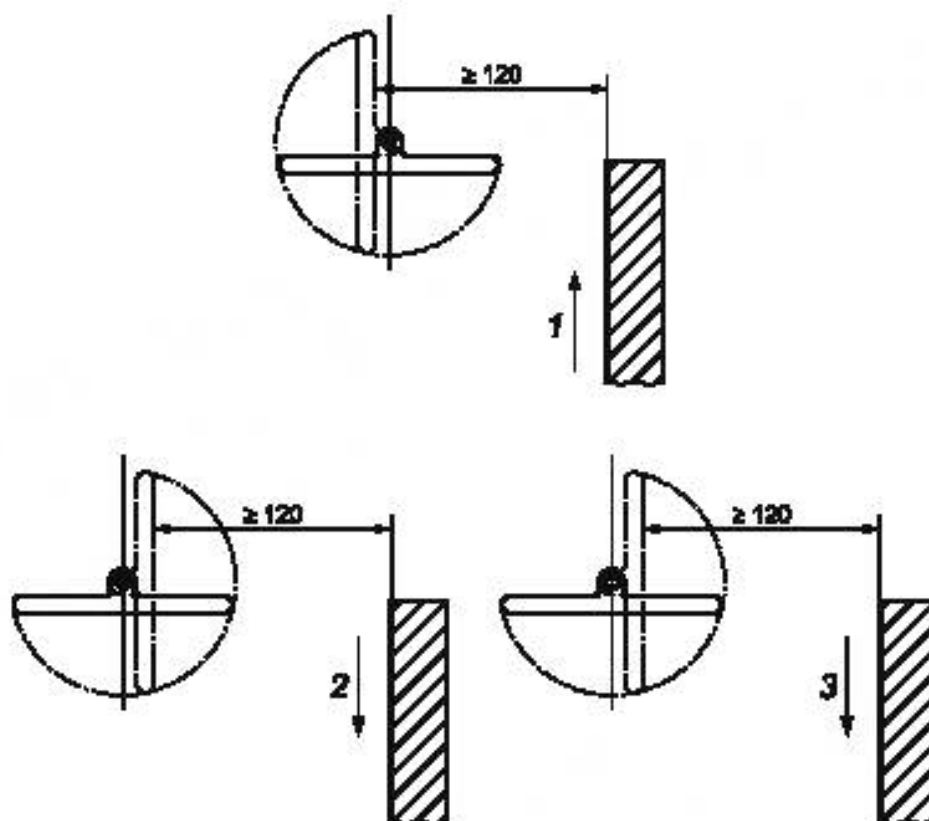
Рисунок 5 — Промежуток между неподвижным краем и осью крепления льюшек
