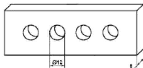
Рисунок 2 — Форма для образцов при испытании на текучесть
