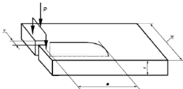
a – Схема испытания
