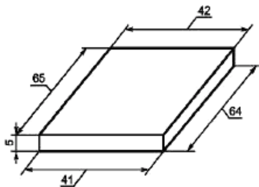
Рисунок 3 — Модель пластины образца
