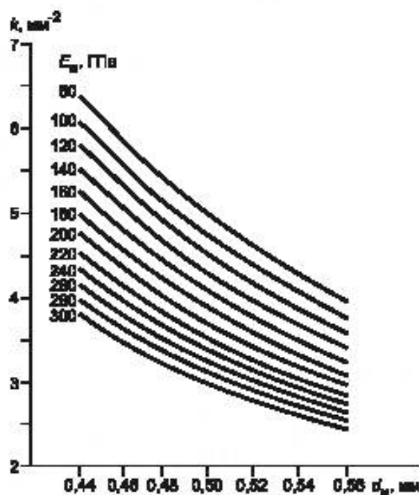
Рисунок 2 — Диаграмма определения коэффициента k как функции толщины металлического каркаса d_m и модуля упругости сплава E_s
