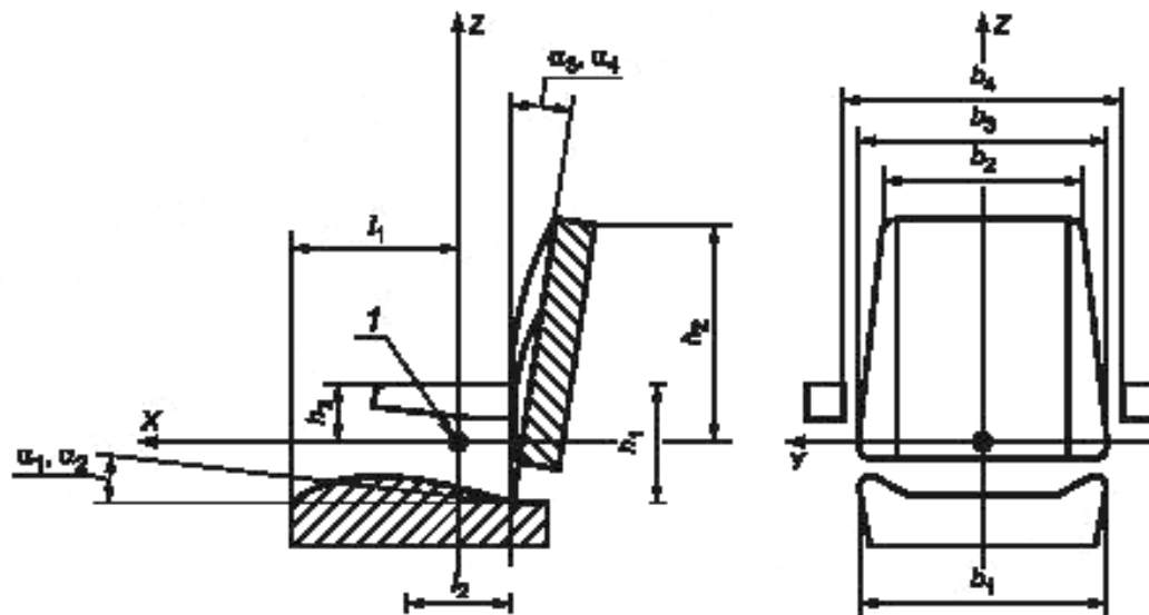
Рисунок 3 — Сиденье оператора
