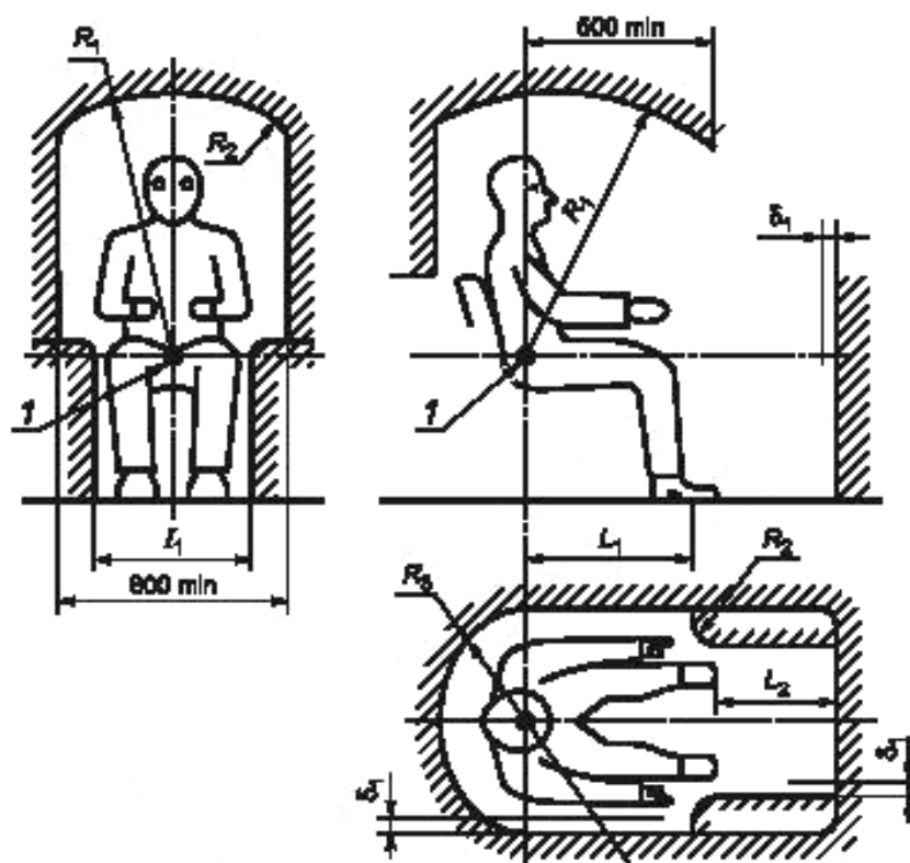
Рисунок 4 — Размеры кабины
