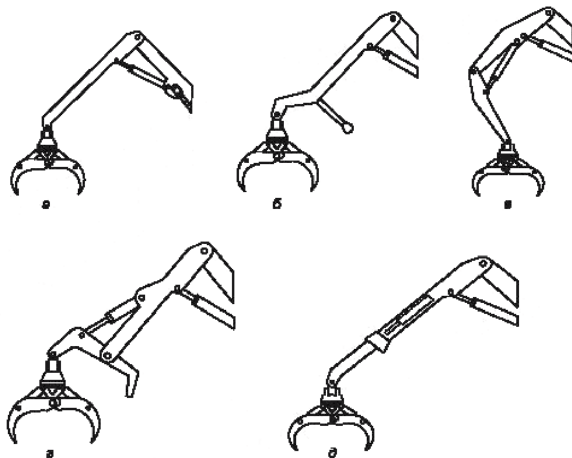
а — стреловое оборудование с прямой рукоятью; б — стреловое оборудование с неподвижным упором на рукояти; в — стреловое оборудование с двухзвенной рукоятью; г — стреловое оборудование с подвижным упором на рукояти; д — стреловое оборудование с телескопической рукоятью
