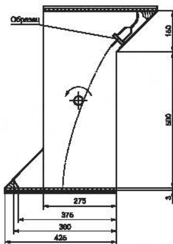
Рисунок 11 — Барабан для испытания соединителей на свободное падение
