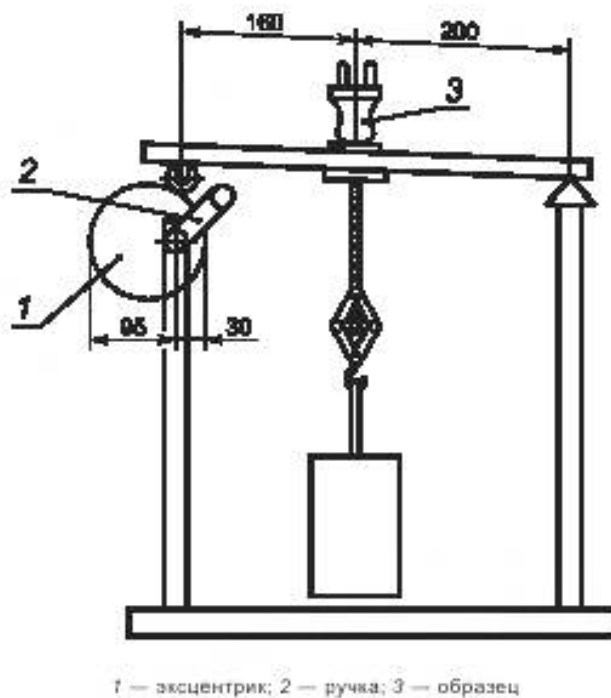
Рисунок 17 — Установка для испытания узла крепления шнура
