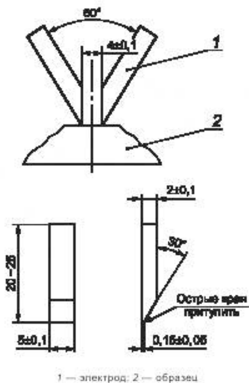
Рисунок 16 — Установка для проверки устойчивости к токам утечки
