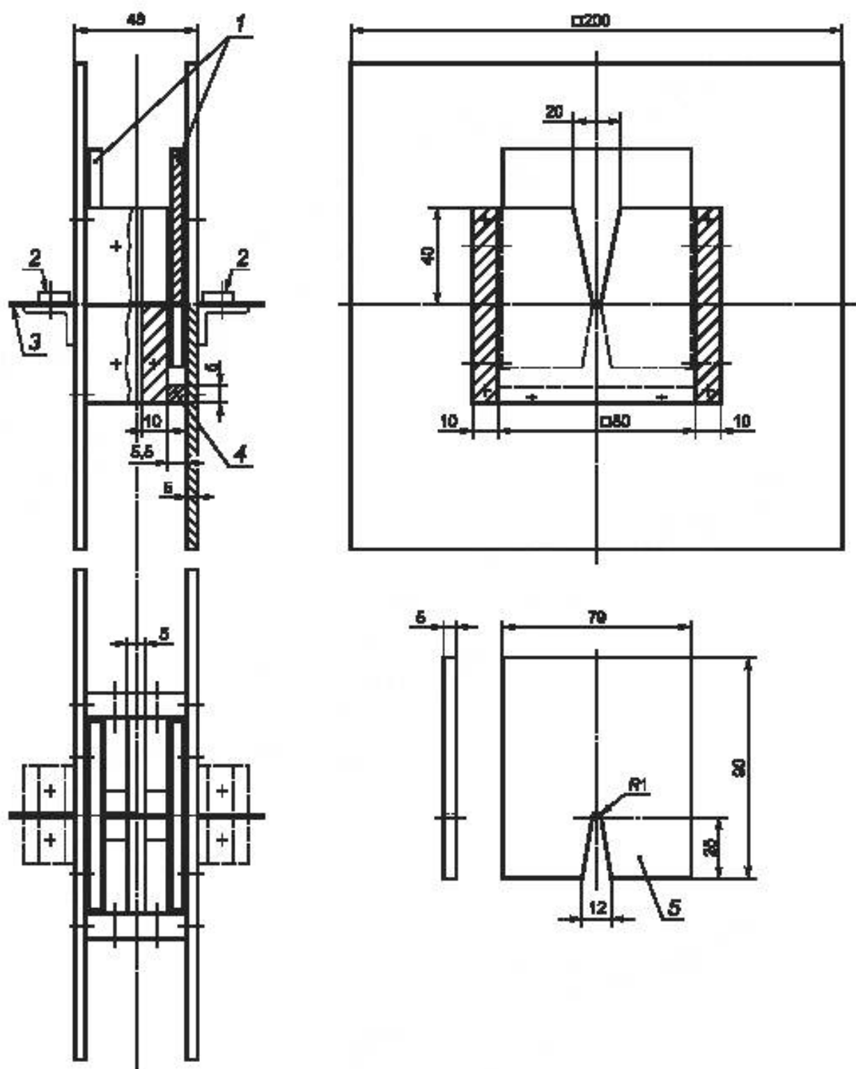
1 — направляющие скользящие пластины; 2 — зажим; 3 — серебряная проволока; 4 — упор для скользящей направляющей пластины; 5 — направляющая скользящая пластина
