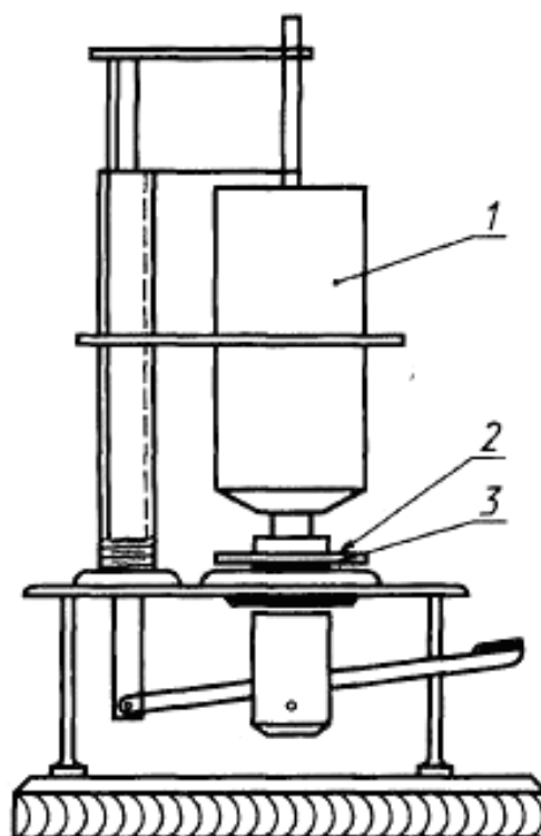
Рисунок 4 — Нагрузочное устройство для определения толщины пленки
