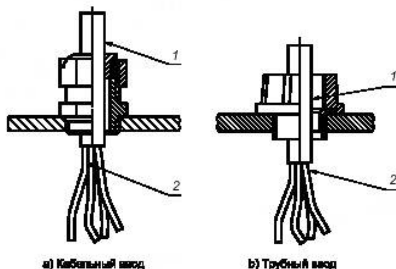
Рисунок 3 — Места ввода и разделки кабеля
