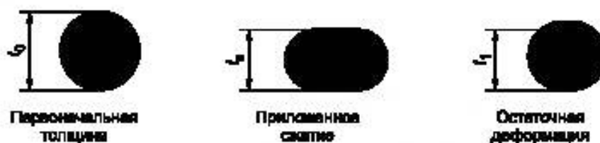
Рисунок 6 — Остаточная деформация при сжатии уплотнительного кольца
