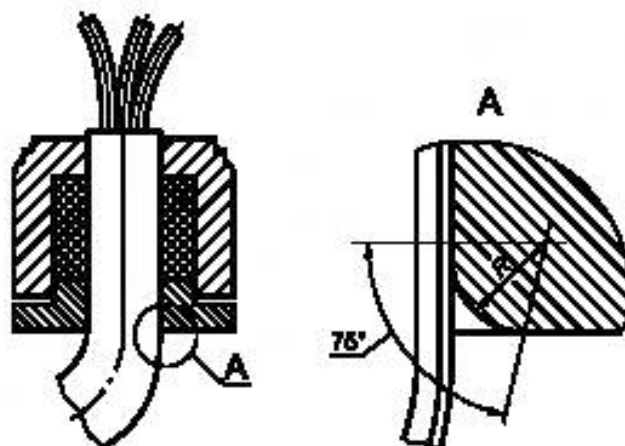
Рисунок A.2 — Скругление кромок в месте ввода гибкого кабеля
