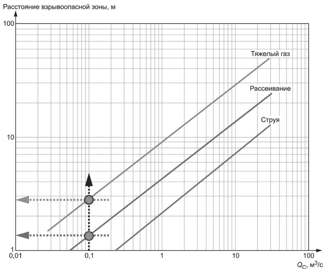
Рисунок Е.2 — Расстояние взрывоопасной зоны (Пример № 1)
