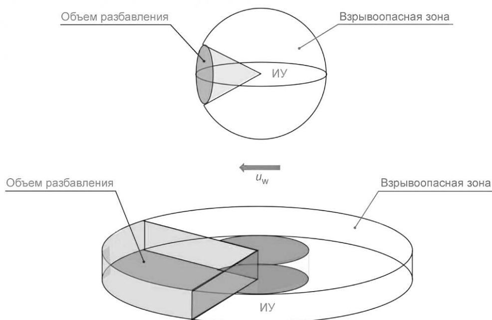
Рисунок 1 — Объем разбавления
