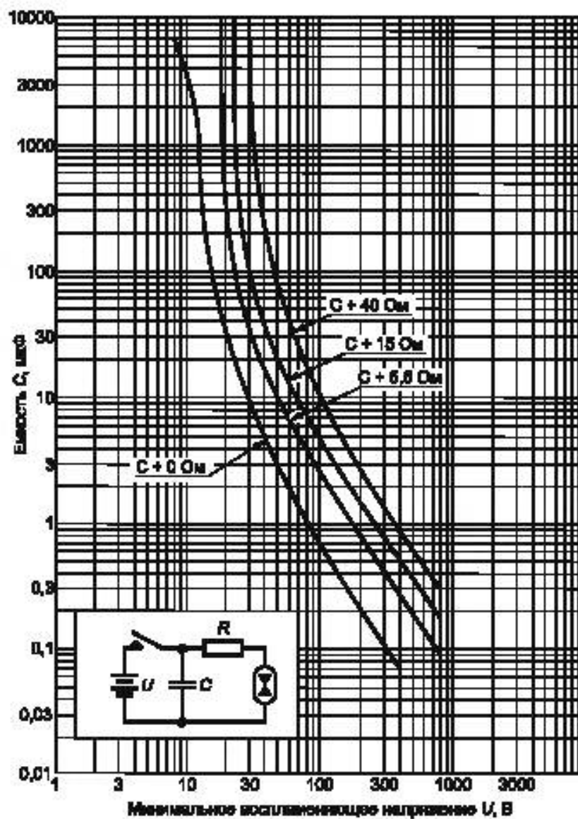
Рисунок А.2 – Емкостные цепи группы I
