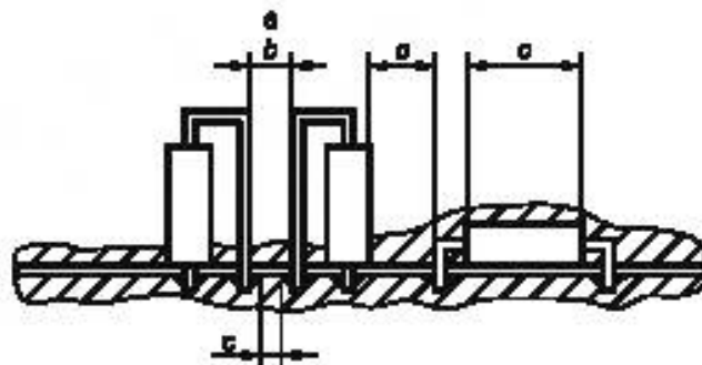
Рисунок б) – Плата с пайкой выступающих выводов разъемов
