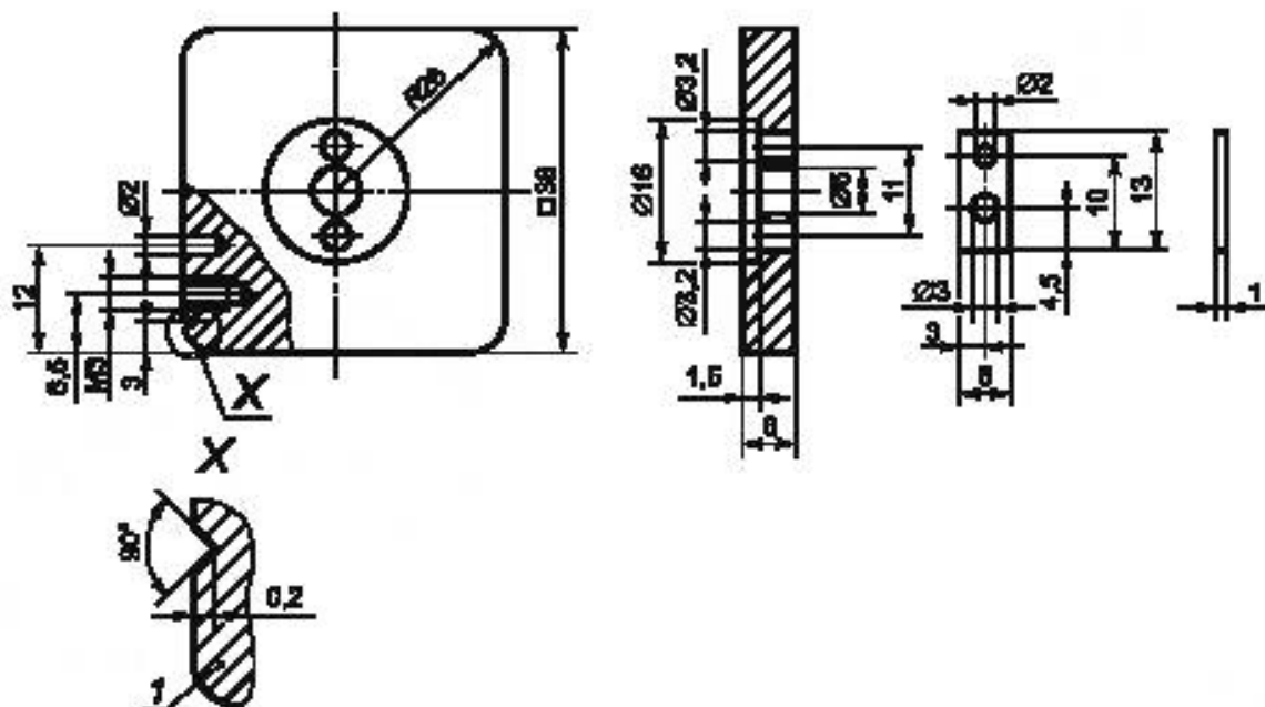
1 – Деталь X. (масштаб 10 : 1)
