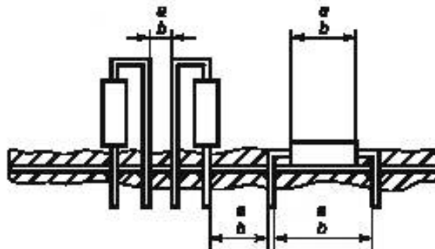
Рисунок б) – Плата с пайкой выступающих выводов разъемов
