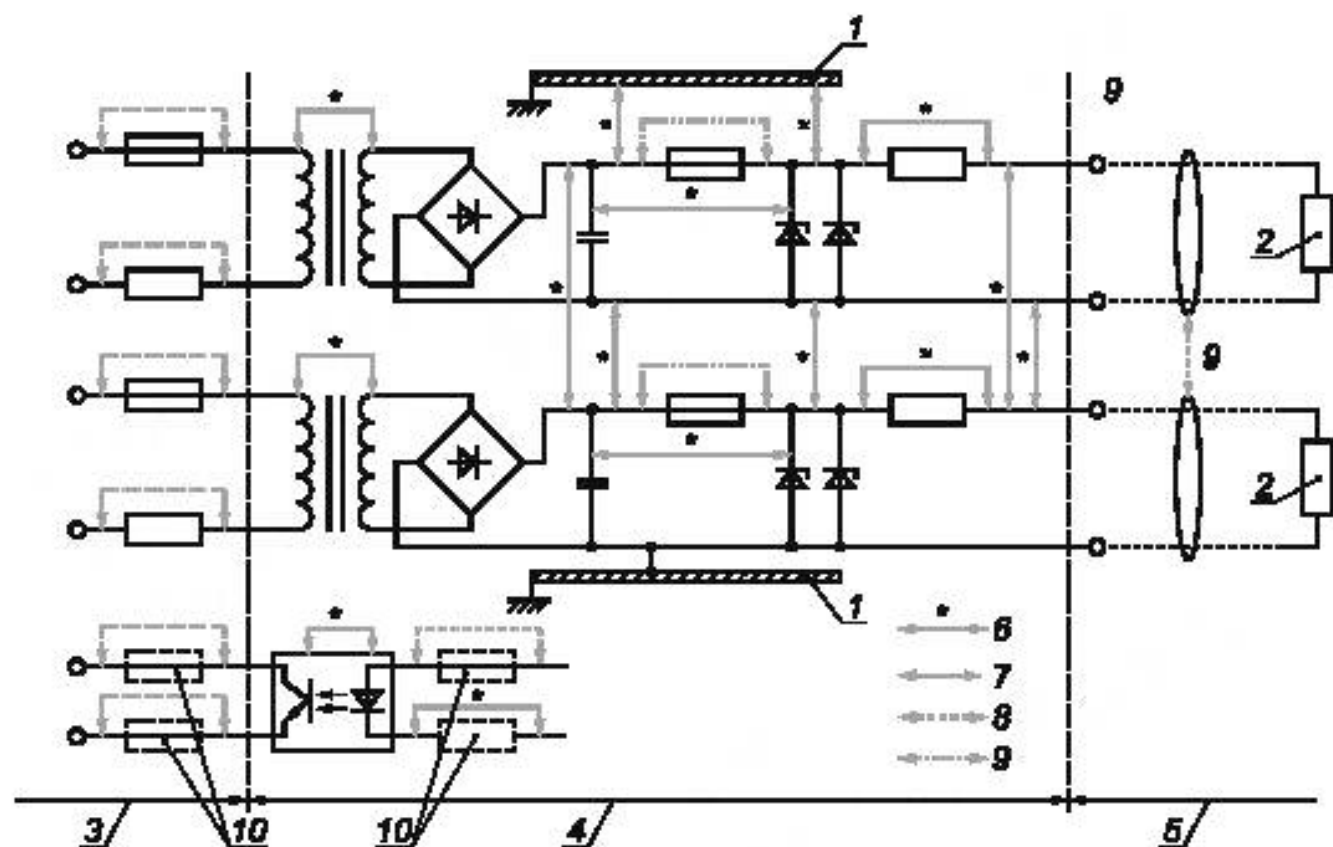
1 – шасси; 2 – нагрузка; 3 – искроопасная цепь с U_m ; 4 – часть искробезопасной цепи, не являющаяся искробезопасной; 5 – искробезопасная цепь; 6 – размеры, определяемые по таблице 5; 7 – размеры, определяемые по общим промышленным стандартам; 8 – размеры в соответствии с 7.3; 9 – размеры в соответствии с 6.2.1 для выходных зажимов между раздельными искробезопасными цепями и между искробезопасными и искроопасными цепями; 10 – если применяются
