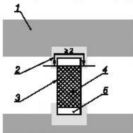
1 – дорожка печатной платы; 2 – паяное сопряжение между подложкой платы и подложкой компонента ( \geq 2 \text{ мм} ); 3 – компонент с неповреждаемым соединением; 4 – подложка для пайки компонента; 5 – размер подложки для пайки печатной платы установлен по данным изготовителя
