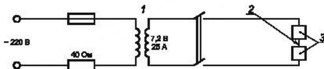
Рисунок В.7 – Устройство для подготовки вольфрамовых проволок методом оплавления
