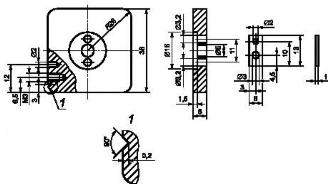
Рисунок В.3 — Держатель проволоки
