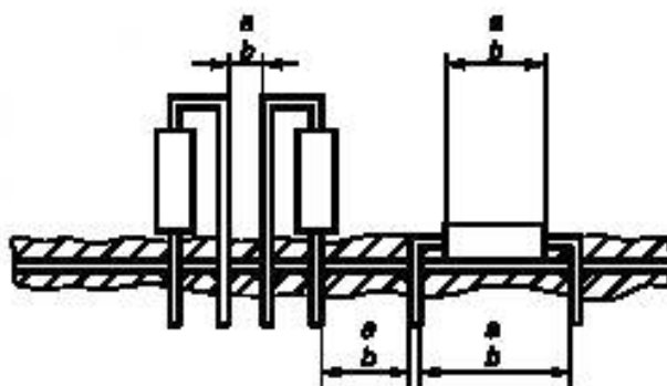
б) Плата с пайкой выступающих выводов резисторов
