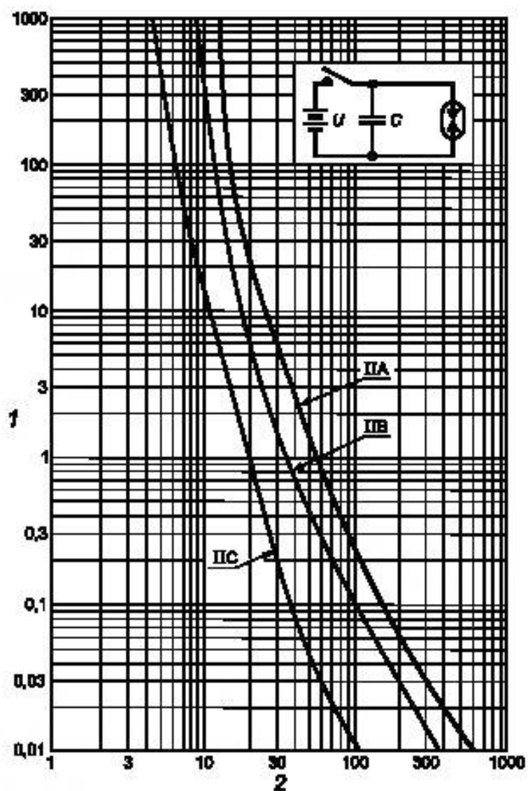
Рисунок А.3 — Емкостные цели группы II
