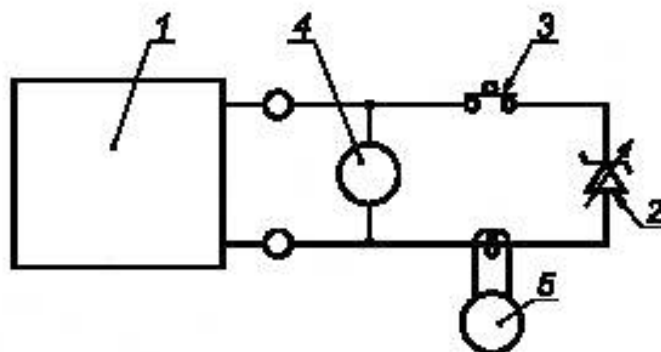
1 — испытуемая цепь; 2 — нагрузка; 3 — ртутный выключатель; 4 — вольтметр высокого сопротивления; 5 — шунт для замера величины тока
