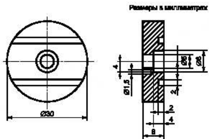
Рисунок В.2 — Кадмиевый контактный диск
