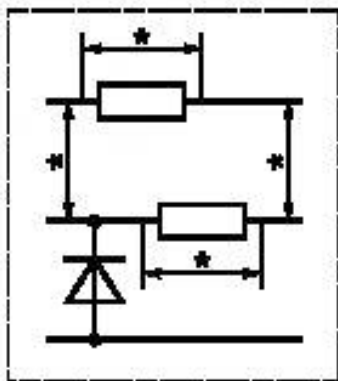
б) Термическая защита
