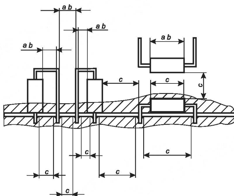
c) Сборка на печатной плате с выводами, сложенными или обрезанными с полным покрытием
