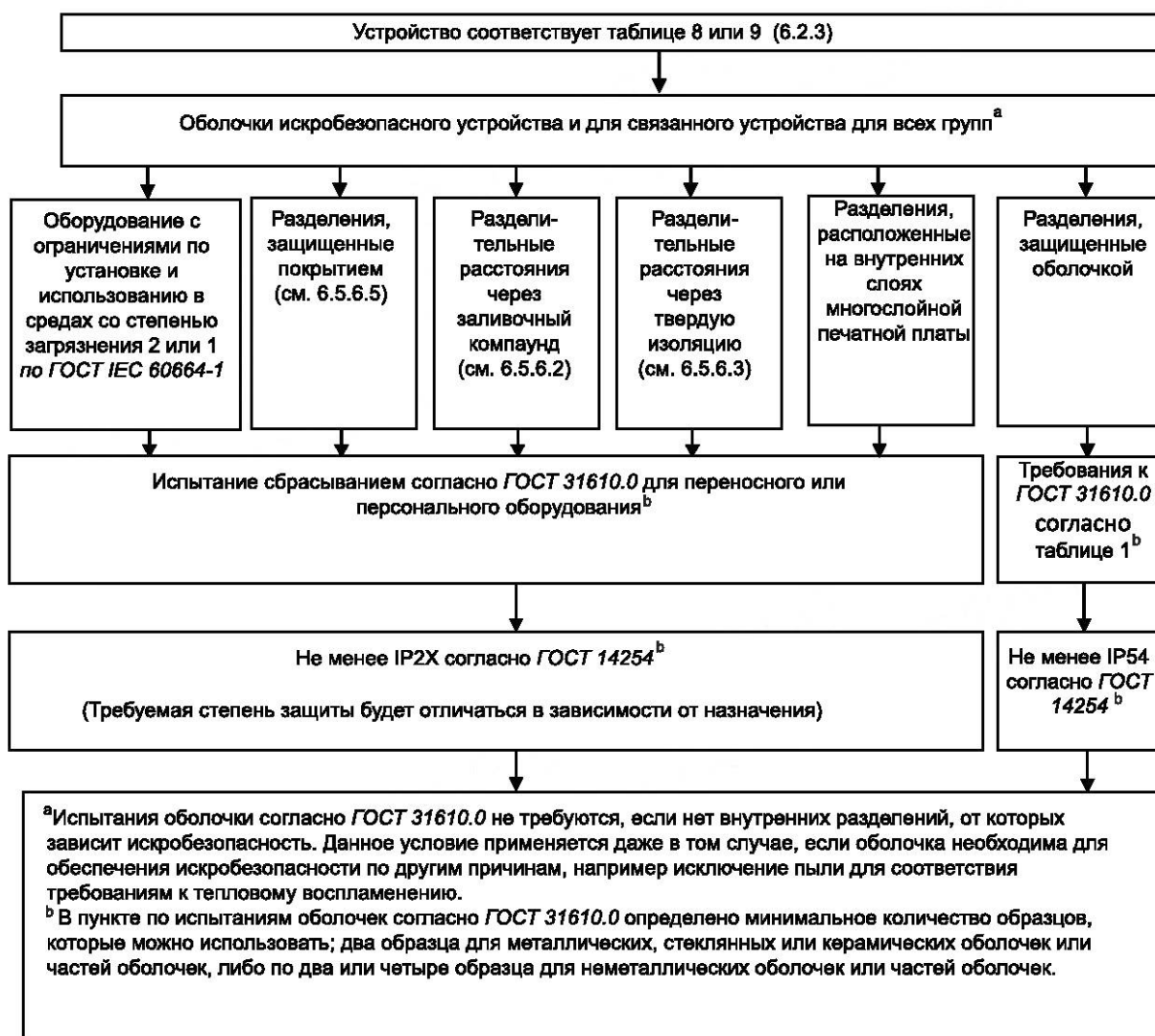
Рисунок 1.2 — Испытания разделительных оболочек или частей оболочек согласно таблице 8 или 9
