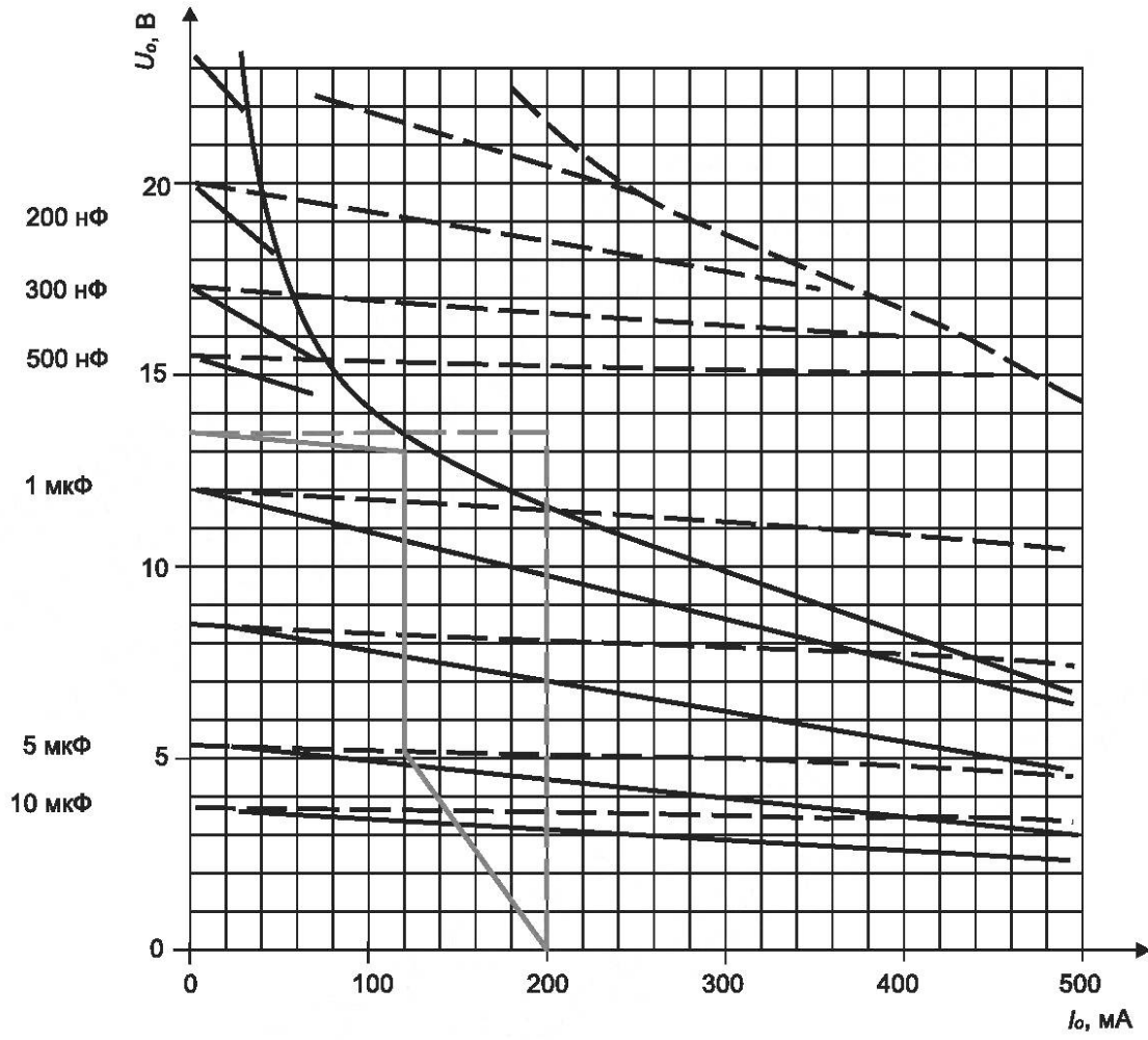
Рисунок G.1 — Примеры выходных характеристик для подгруппы IIC
