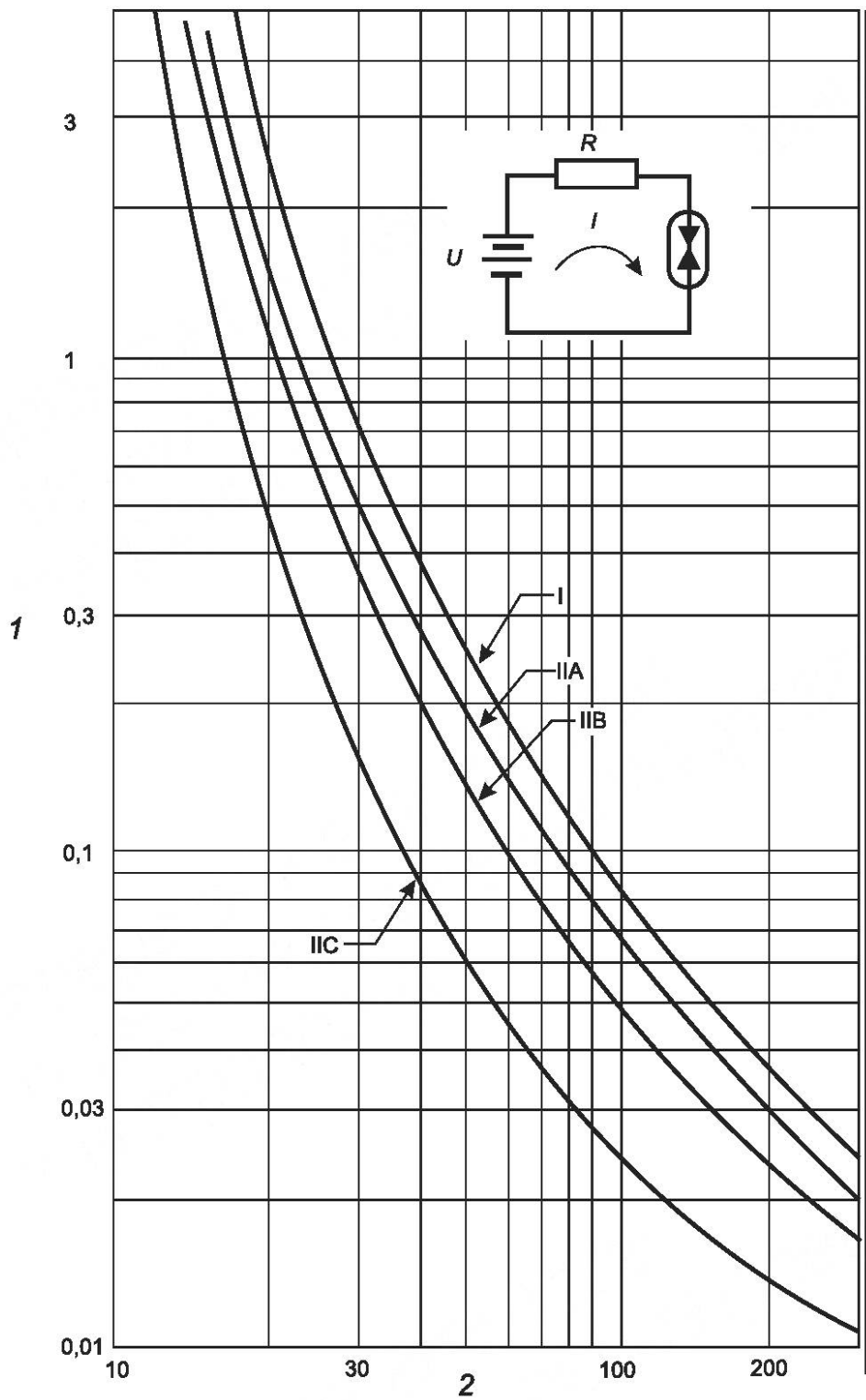
Рисунок А.1 — Омические цепи
