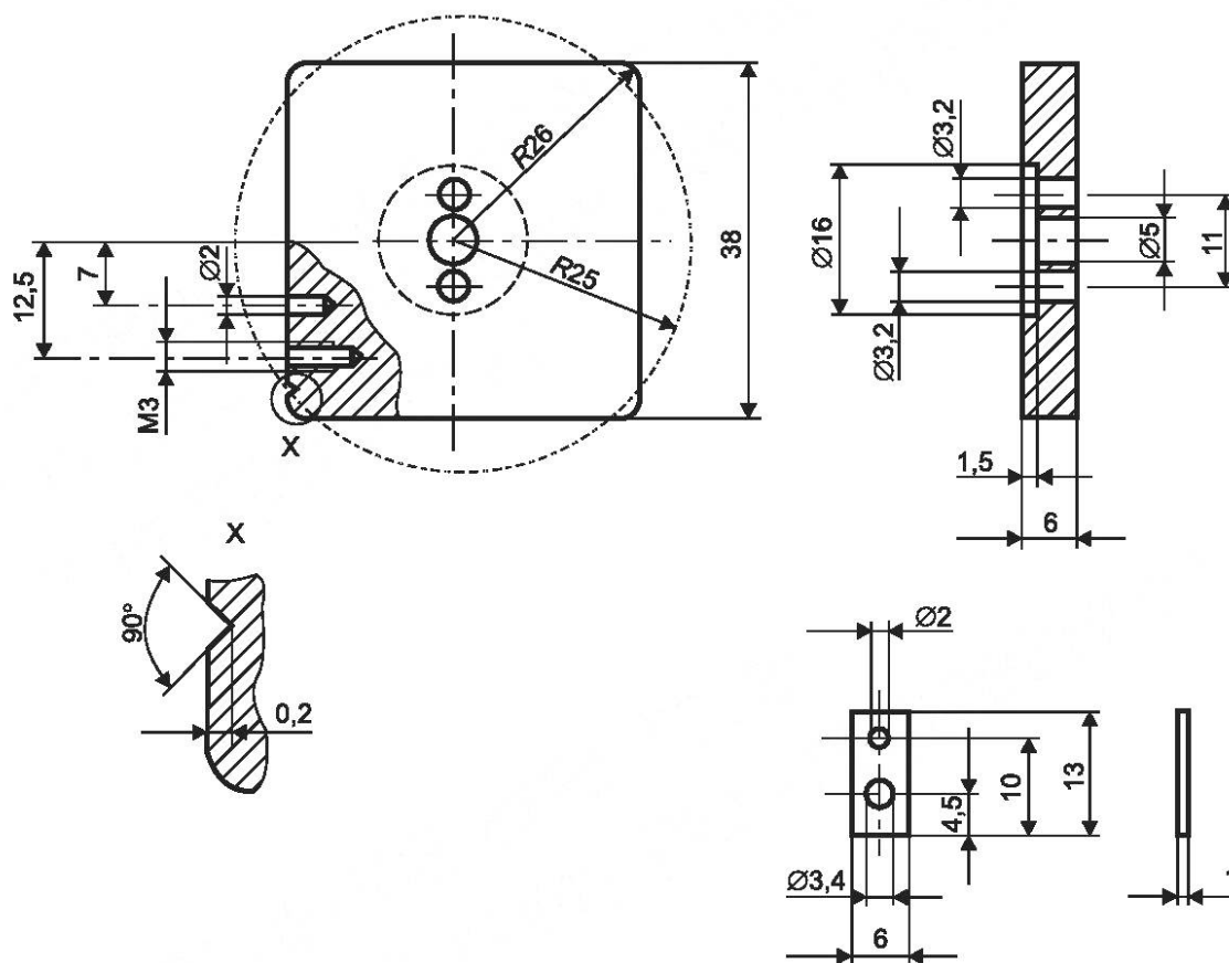
Рисунок В.3 — Держатель проволоочек
