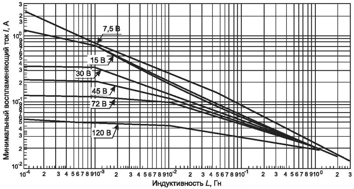
Рисунок A.4c — Индуктивные цепи подгруппы IIB
