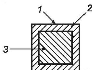
1 — свободная поверхность, внешняя стенка; 2 — компаунд; 3 — компонент — компаунд не должен проникать в компонент
