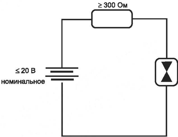
Рисунок 12 — Пример простой резистивной цепи
