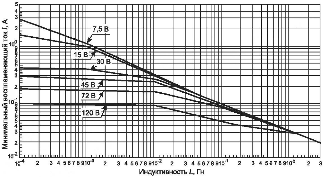
Рисунок A.4b — Индуктивные цепи подгруппы IIA
