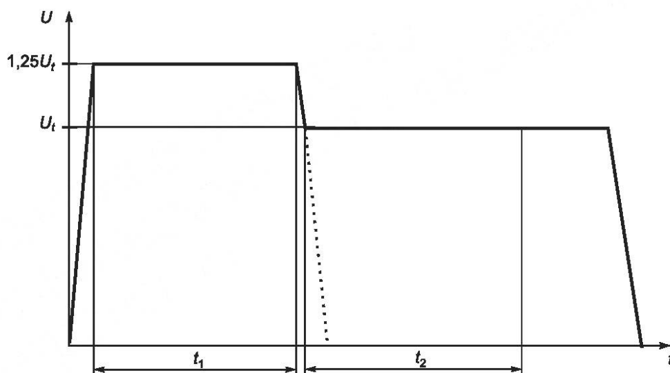
Рисунок 16 — Испытательное напряжение
