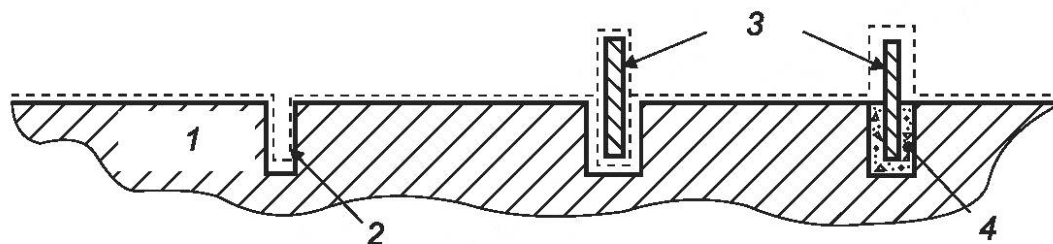
1 — подложка; 2 — бороздка; 3 — перегородка; 4 — клей
