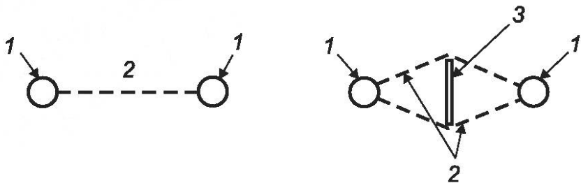
1 — проводник; 2 — электрический зазор; 3 — перегородка
