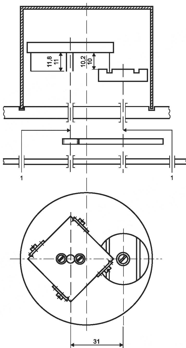
Рисунок В.1 — Искрообразующее устройство для испытания искробезопасных цепей
