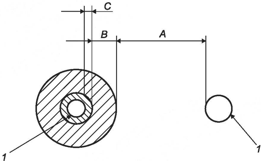
1 — проводник; А — электрический зазор; В — разделительное расстояние через компаунд; С — разделительное расстояние через твердую изоляцию
