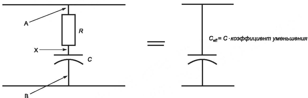
Рисунок 14 — Эффективная емкость
