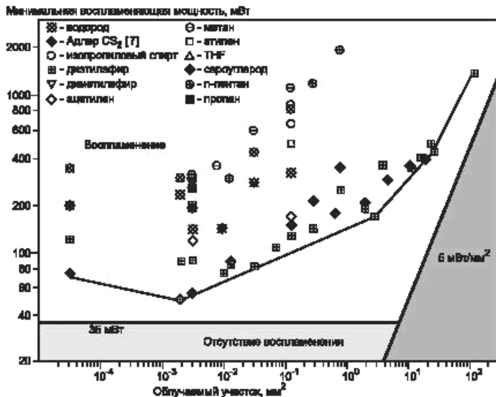
Рисунок В.1 — Минимальная воспламеняющая мощность излучения с инертным поглотителем в качестве облучаемого материала ( \alpha_{1064 \text{ нм}} = 83\% , \alpha_{2025 \text{ нм}} = 93 ) при непрерывном облучении в волновом диапазоне 1064 нм
