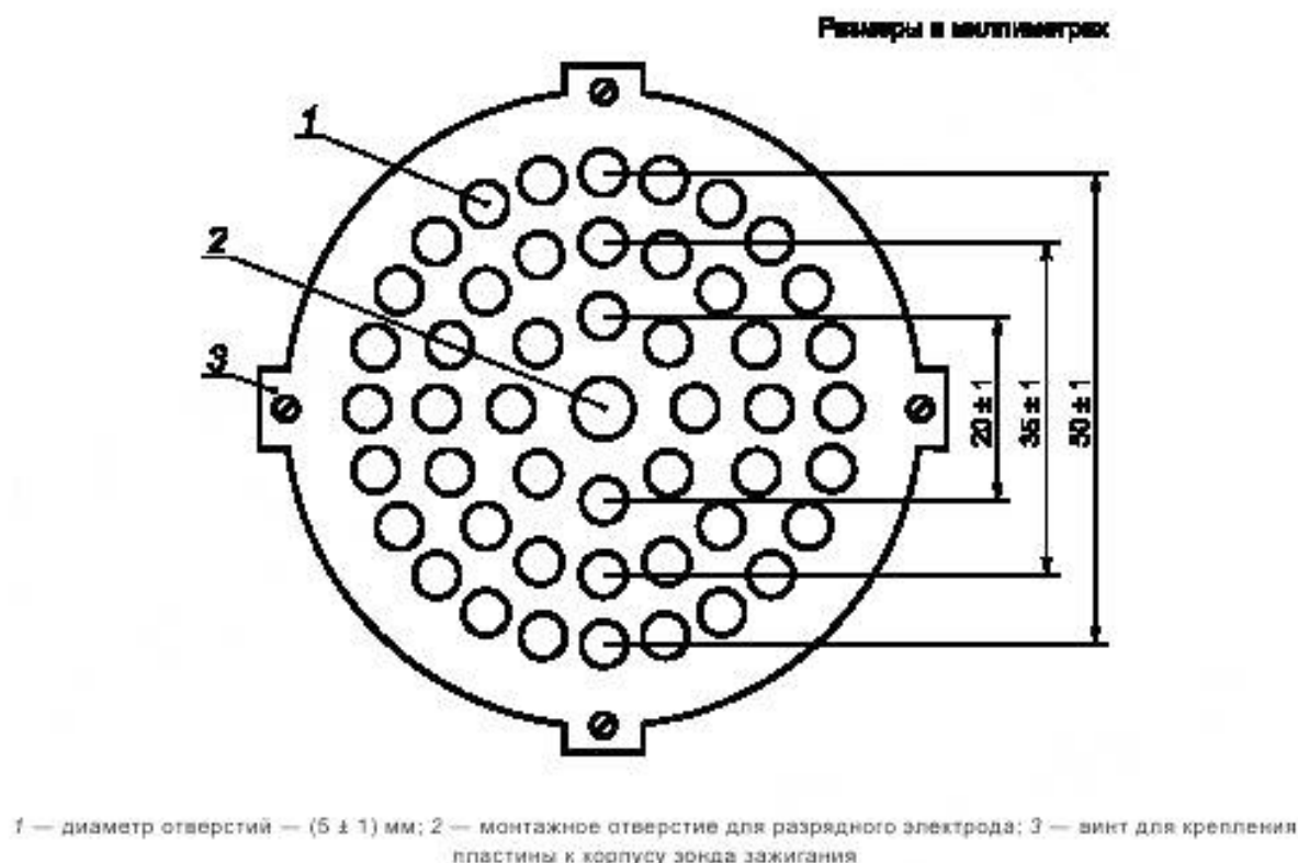
Рисунок G.5 — Перфорированная металлическая пластина зонда зажигания
