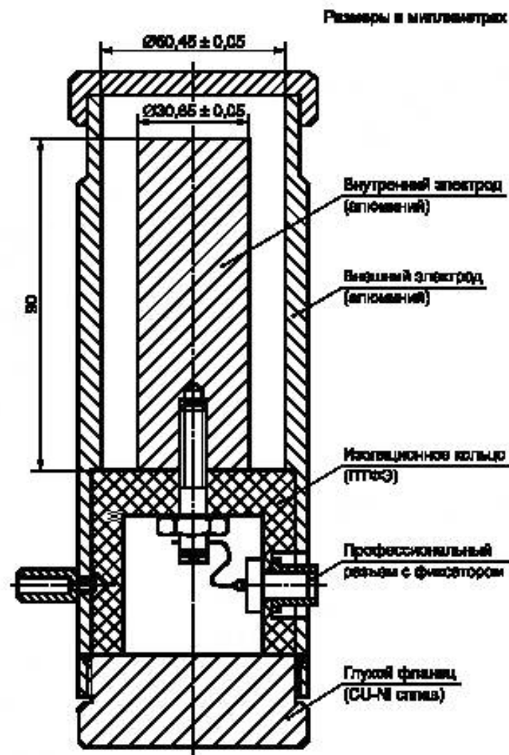
Рисунок G.3 — Ячейка для измерения проводимости жидкости
