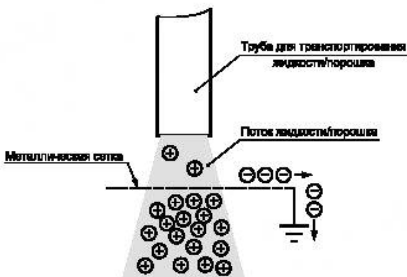
Рисунок 5 — Опасность размещения заземленного проводника в непроводящем потоке.
