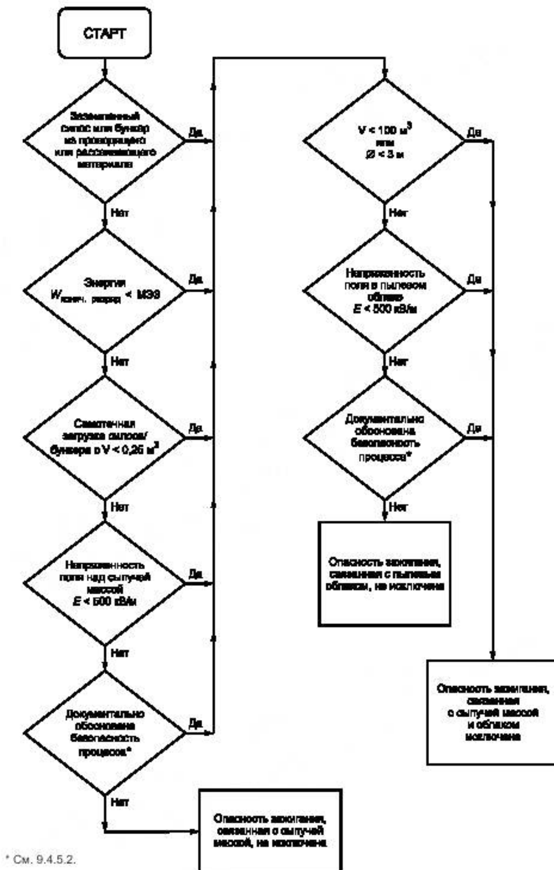
Рисунок 2 — Блок-схема: оценка сыпучего материала с 1 \text{ МОм м} < \rho \leq 10 \text{ ГОм м}
