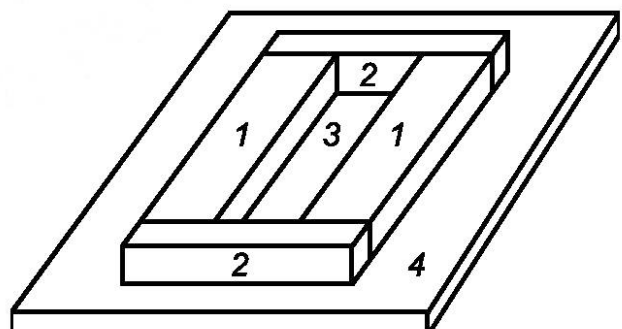
Рисунок 2 — Ячейка для измерения удельного сопротивления порошка
